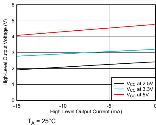
图 5-7. 高电平输出电压与高电平输出电流之间的关系
