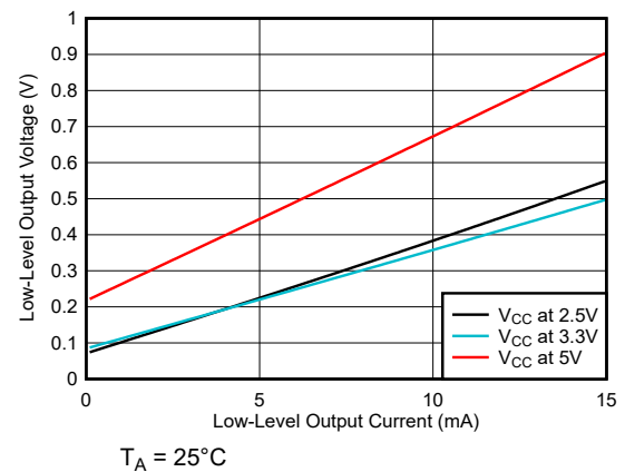
图 5-8. 低电平输出电压与低电平输出电流之间的关系
