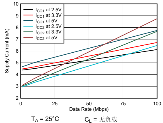
图 5-4. ISO7741Tx-Q1 电源电流与数据速率之间的关系 (无负载)
