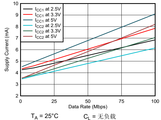
图 5-6. ISO7742Tx-Q1 电源电流与数据速率之间的关系 (无负载)
