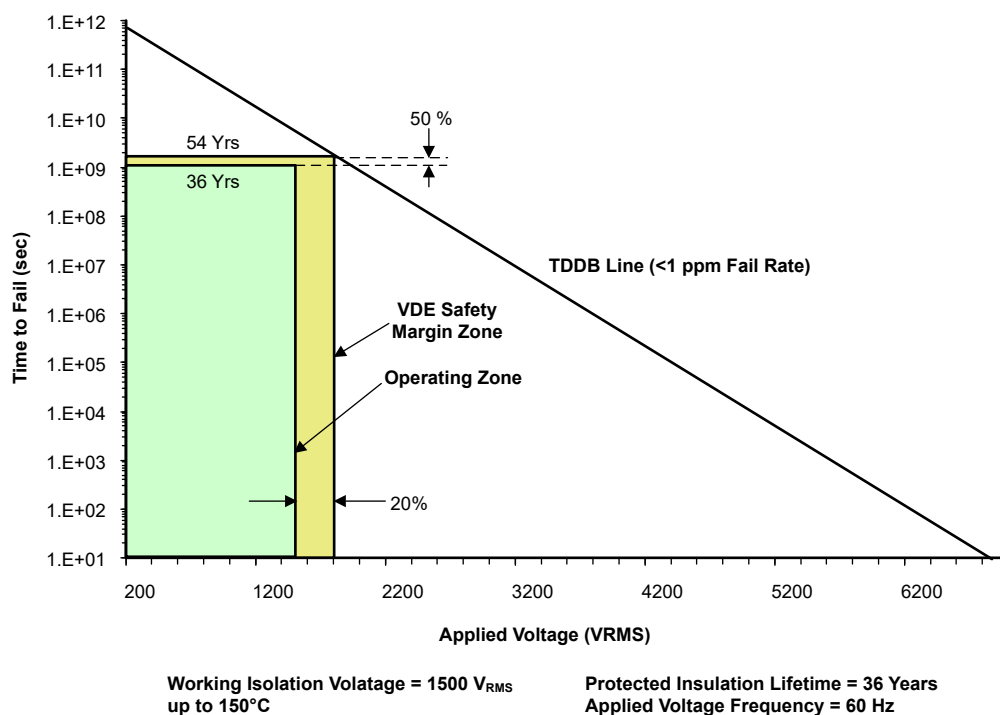
图 8-7. 绝缘寿命预测数据
