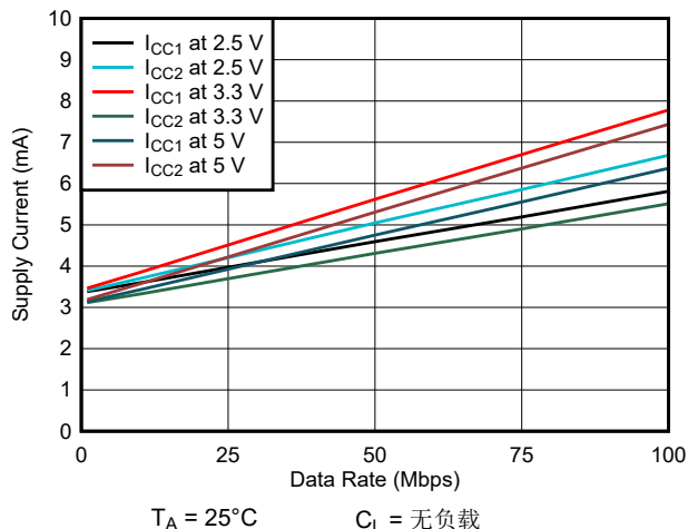
图 5-12. ISO7742-Q1 电源电流与数据速率间的关系 (无负载)
