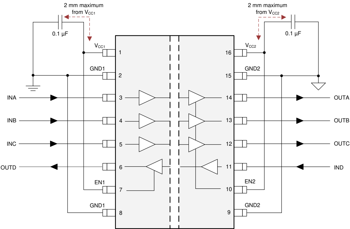
图 8-2. 典型 ISO7741E-Q1 电路组装
