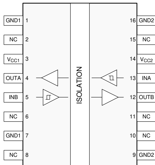
图 5-2. ISO7721-Q1 DW 封装 16 引脚 SOIC 顶视图
