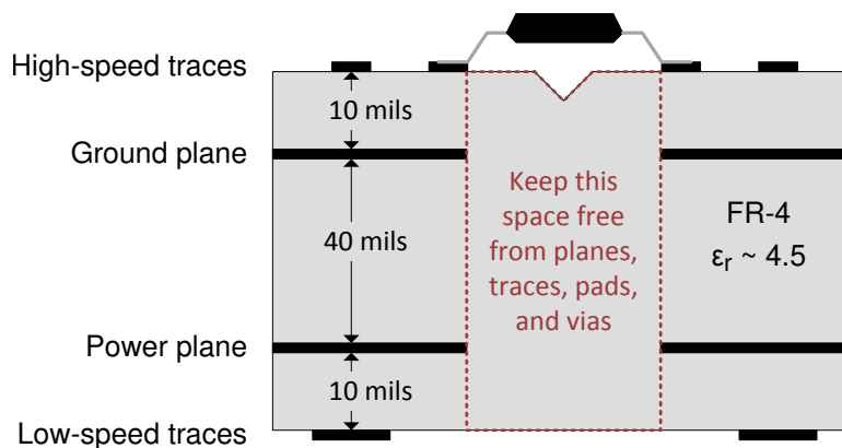
图 25-6. Layout Example
