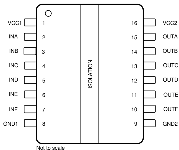
图 5-1. ISO6760-Q1 DW Package 16-Pin SOIC-WB Top View
