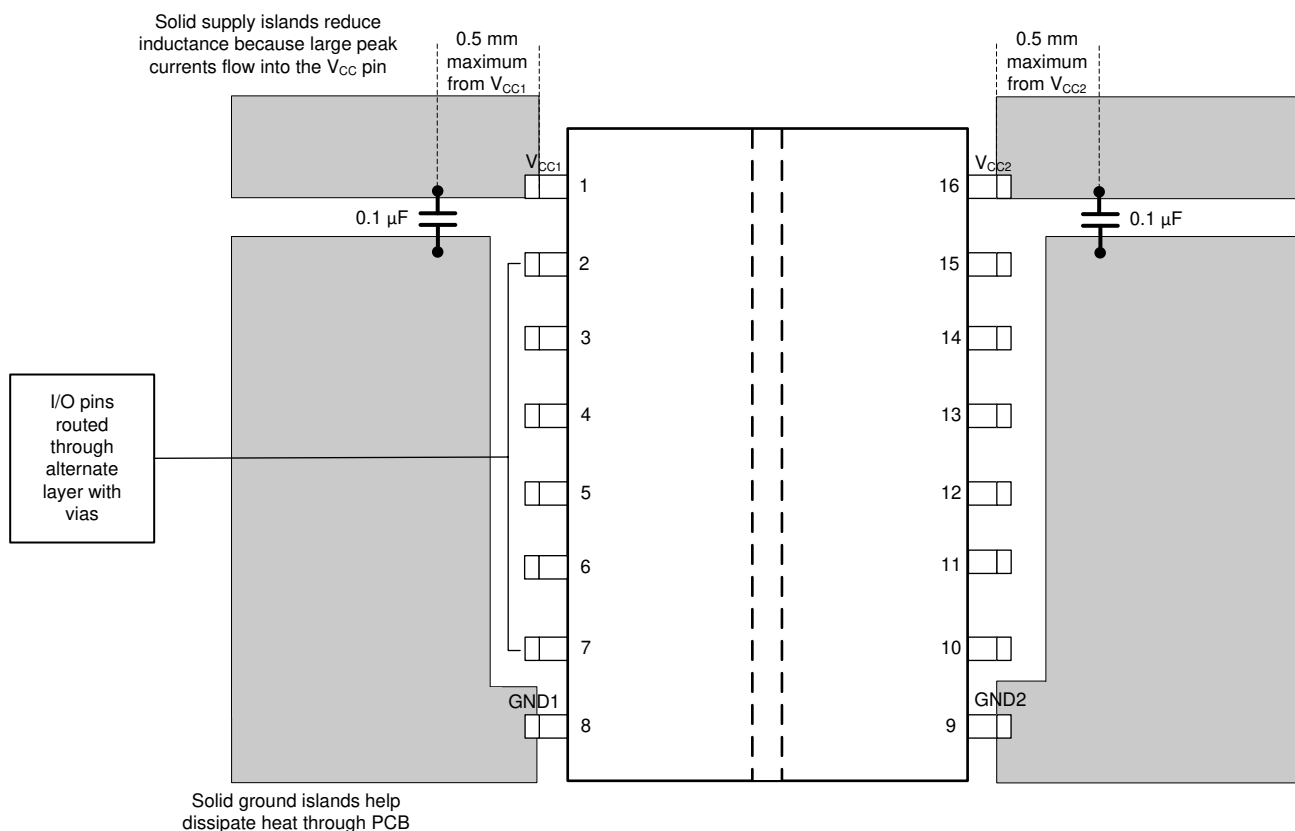
图 11-1. Layout Example
