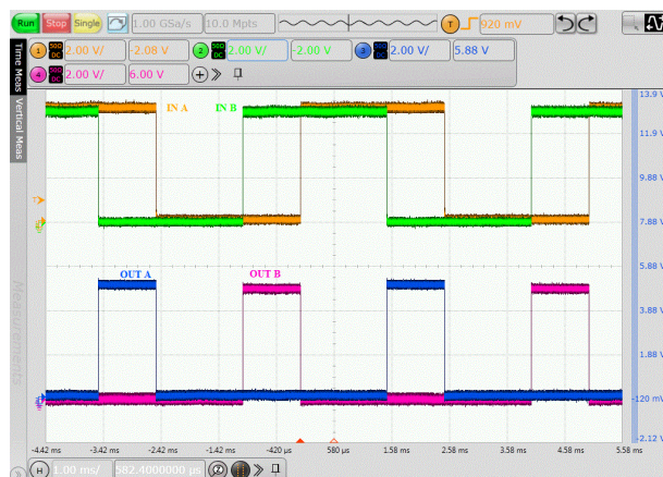
图 9-3. ISO6760L 互锁图
