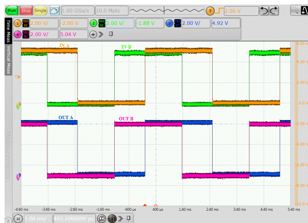
图 9-4. ISO6760 ( 不带互锁的器件 ) 图
