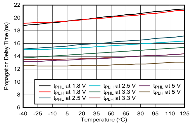
图 6-7. 传播延迟时间与自然通风条件下的温度间的关系
