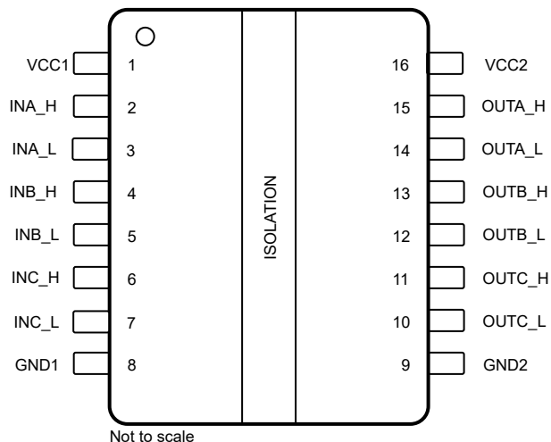
图 5-1. ISO6760L DW 封装 16 引脚 SOIC-WB 顶视图
