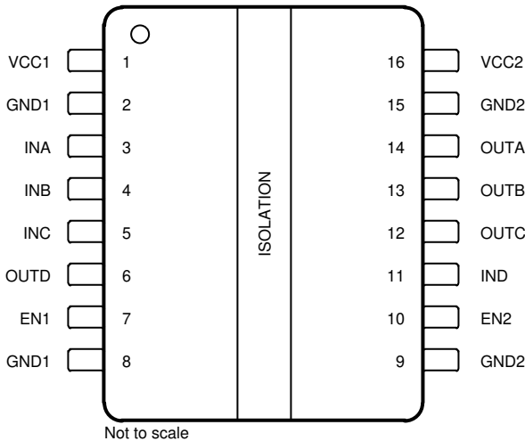
图 4-2. ISO6741-Q1 DW 封装 16 引脚 SOIC-WB 顶视图
