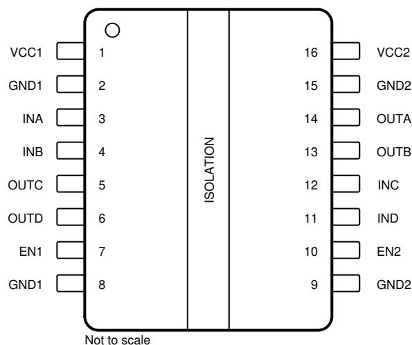
图 4-3. ISO6742-Q1 DWW 封装 16 引脚 SOIC-Extra-WB、SOIC-WB 顶视图
