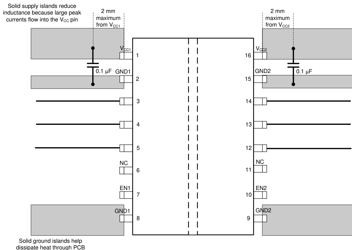
图 11-1. Layout Example
