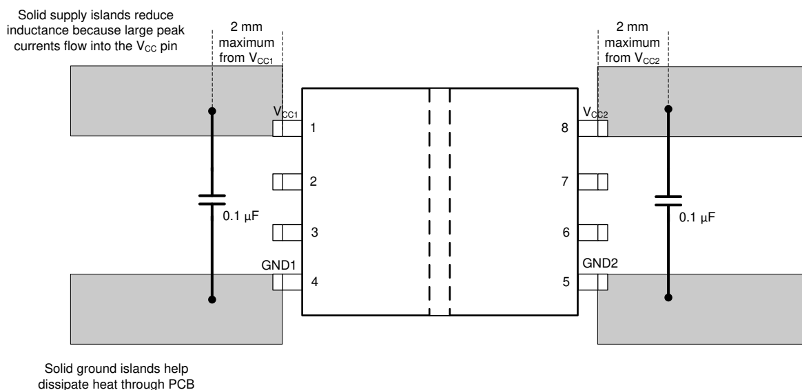
图 12-1. Layout Example
