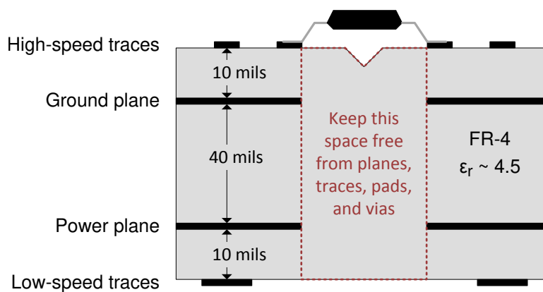
图 8-7. 布局示例 PCB 横截面
