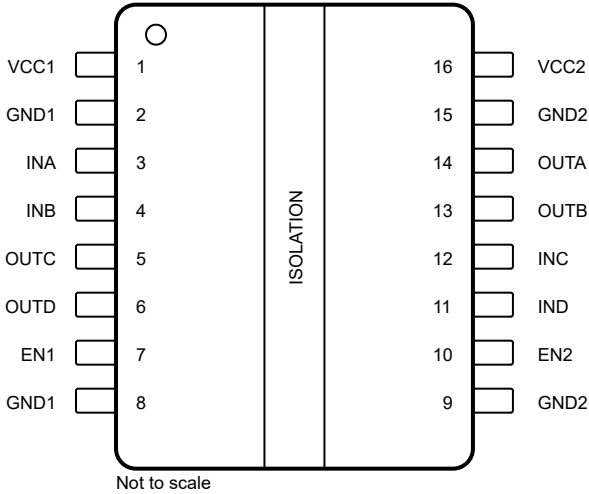
图 4-3. ISO6542 和 ISO6542F 顶视图
