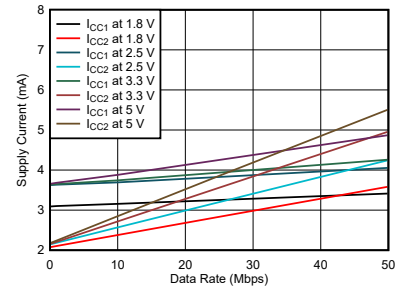
图 5-2. ISO6540 或 ISO6540F 电源电流与数据速率间的关系 (无负载)
