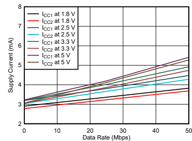
图 5-4. ISO6541 或 ISO6541F 电源电流与数据速率间的关系 (无负载)
