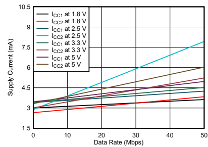
图 5-2. ISO6540 或 ISO6540F 电源电流与数据速率间的关系 (无负载)
