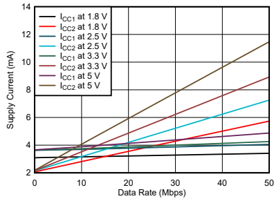
图 5-1. ISO6540 或 ISO6540F 电源电流与数据速率间的关系 (15pF 负载)
