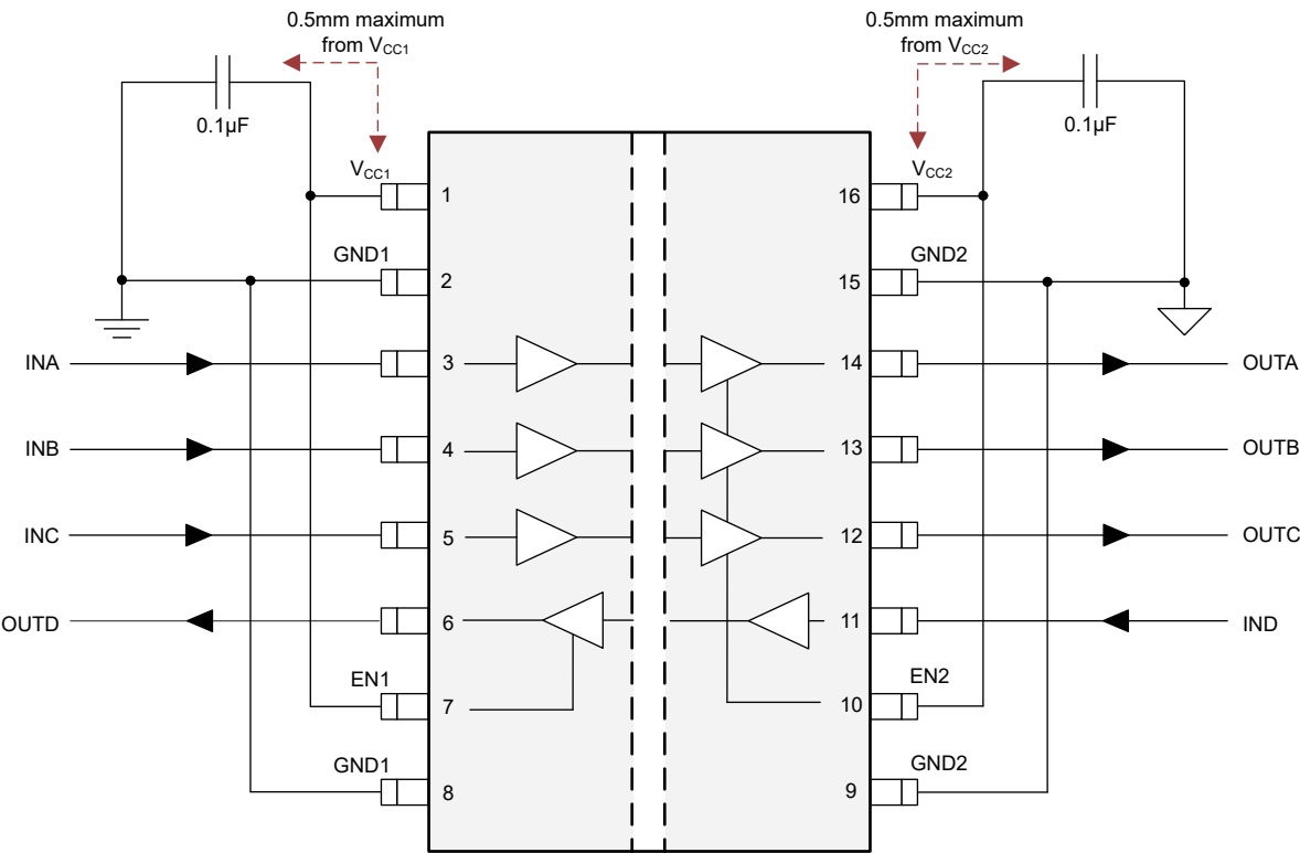
图 8-2. 典型 ISO654x 电路
