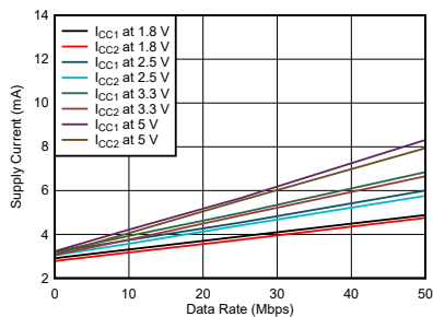
图 5-3. ISO6541 或 ISO6541F 电源电流与数据速率间的关系 (15pF 负载)
