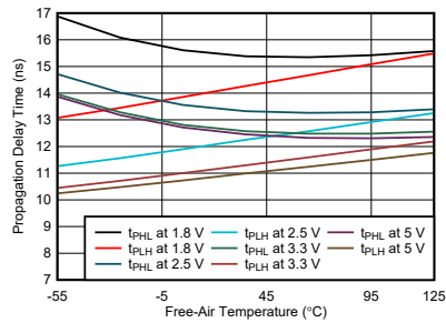
图 5-10. 传播延迟时间与自然通风条件下的温度间的关系
