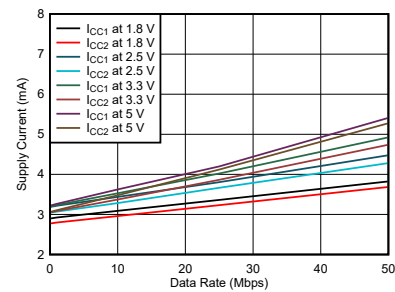
图 5-4. ISO6541-Q1 或 ISO6541F-Q1 电源电流与数据速率间的关系 (无负载)
