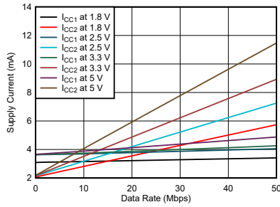
图 5-1. ISO6540-Q1 或 ISO6540F-Q1 电源电流与数据速率间的关系 (15pF 负载)
