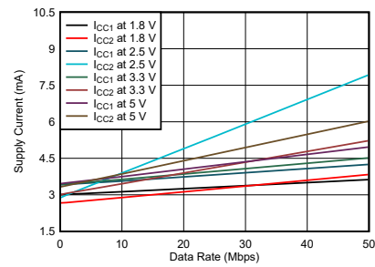
图 5-2. ISO6540-Q1 或 ISO6540F-Q1 电源电流与数据速率间的关系 (无负载)
