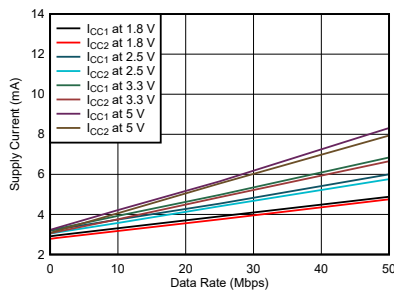
图 5-3. ISO6541-Q1 或 ISO6541F-Q1 电源电流与数据速率间的关系 (15pF 负载)
