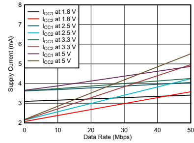
图 5-2. ISO6540-Q1 或 ISO6540F-Q1 电源电流与数据速率间的关系 (无负载)
