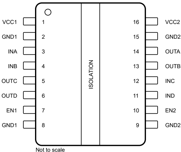
图 4-3. ISO6542-Q1 和 ISO6542F-Q1 顶视图
