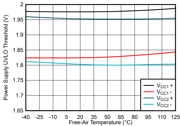
图 6-9. 电源欠压阈值与自然通风条件下的温度间的关系
