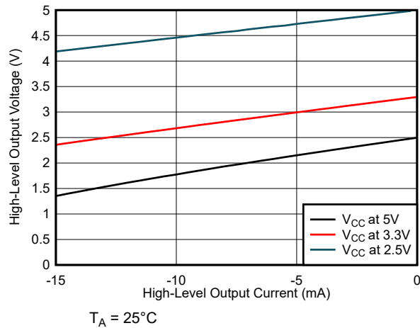
图 6-7. 高电平输出电压与高电平输出电流间的关系
