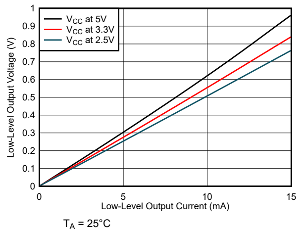
图 6-8. 低电平输出电压与低电平输出电流间的关系
