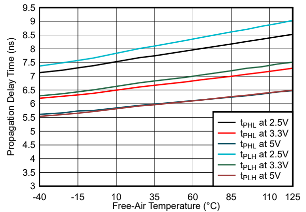
图 6-10. 传播延迟时间与自然通风条件下的温度间的关系
