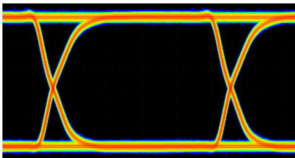
图 9-4. 100Mbps PRBS 2 16 – 1、3.3V 和 25°C 下的 ISO646x 眼图
