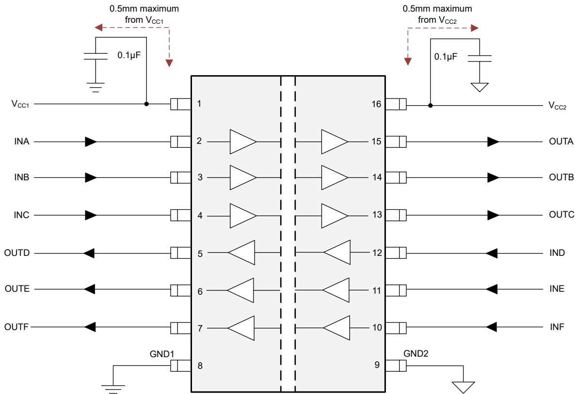
图 9-2. 典型 ISO646x 电路
