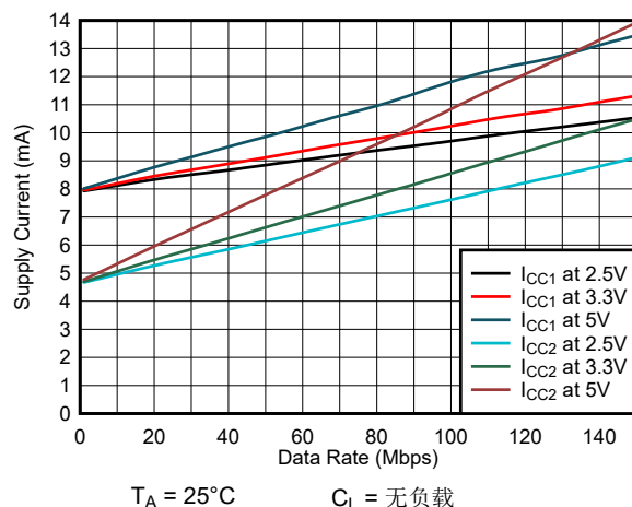
图 6-4. ISO6462 或 ISO6462F 电源电流与数据速率间的关系 (无负载)
