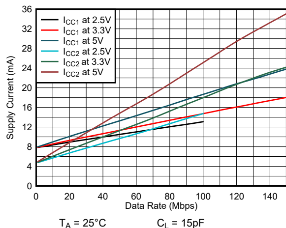
图 6-3. ISO6462 或 ISO6462F 电源电流与数据速率间的关系 (15pF 负载)
