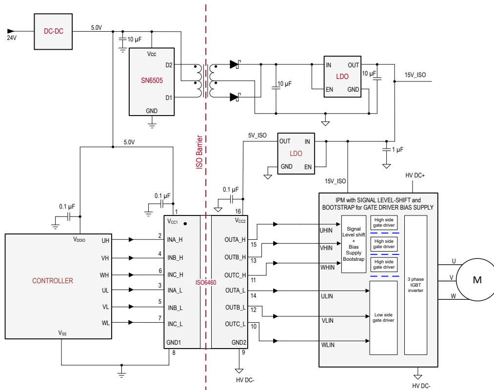
图 9-1. 6 通道典型应用
