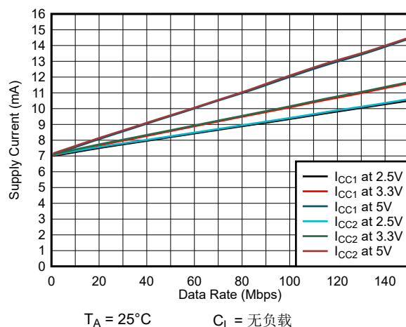
图 6-6. ISO6463 或 ISO6463F 电源电流与数据速率间的关系 (无负载)
