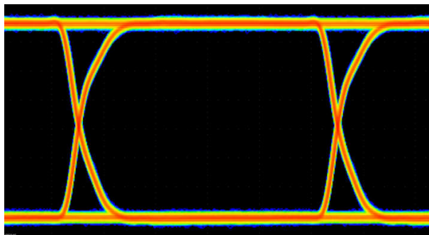
图 9-4. 100Mbps PRBS 2 16 – 1、3.3V 和 25°C 下的 ISO646x 眼图
