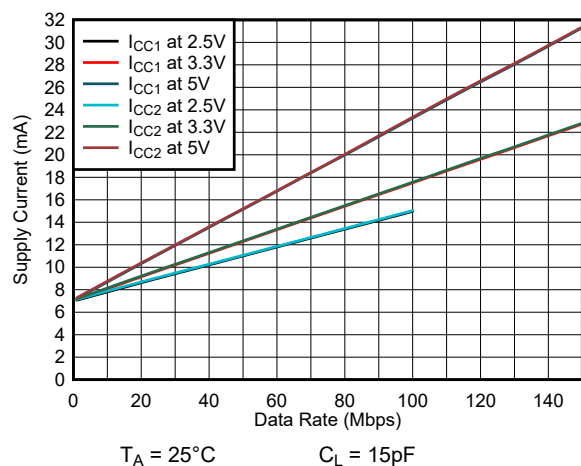
图 6-5. ISO6463 或 ISO6463F 电源电流与数据速率间的关系 (15pF 负载)
