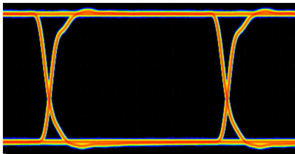
图 9-3. 100Mbps PRBS 2 16 – 1、5V 和 25°C 下的 ISO646x 眼图
