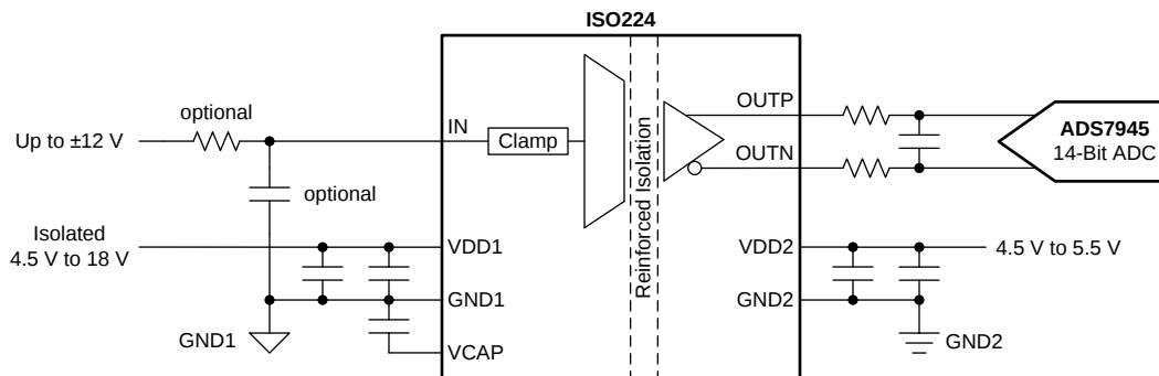
简化原理图
