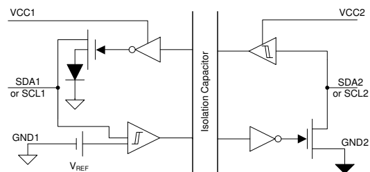
简化的隔离式双向数据通道原理图
