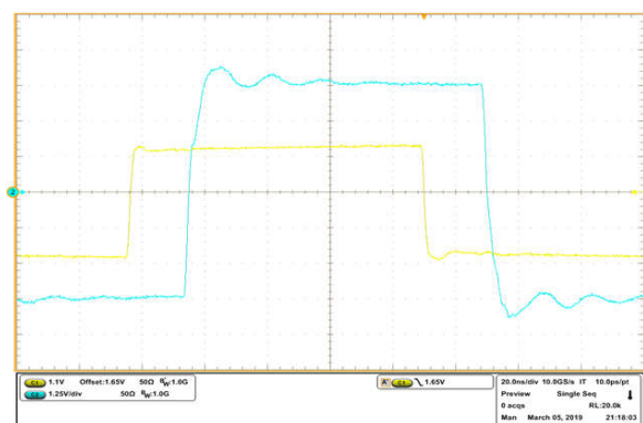
图 7-31. ISO145x 驱动器传播延迟
