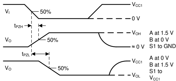
图 8-10. 接收器启用和禁用时间
