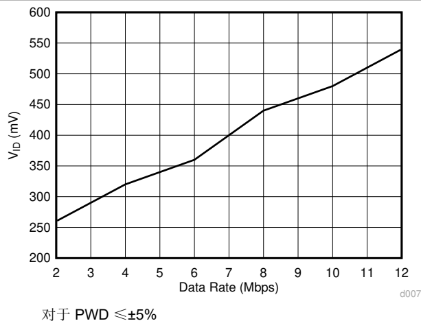
图 7-27. ISO143x 接收器 V_{ID} 与信令速率间的关系
