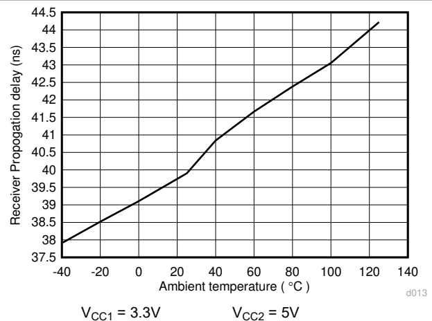
图 7-26. ISO145x 接收器传播延迟 (ns) 与温度 (C) 间的关系
