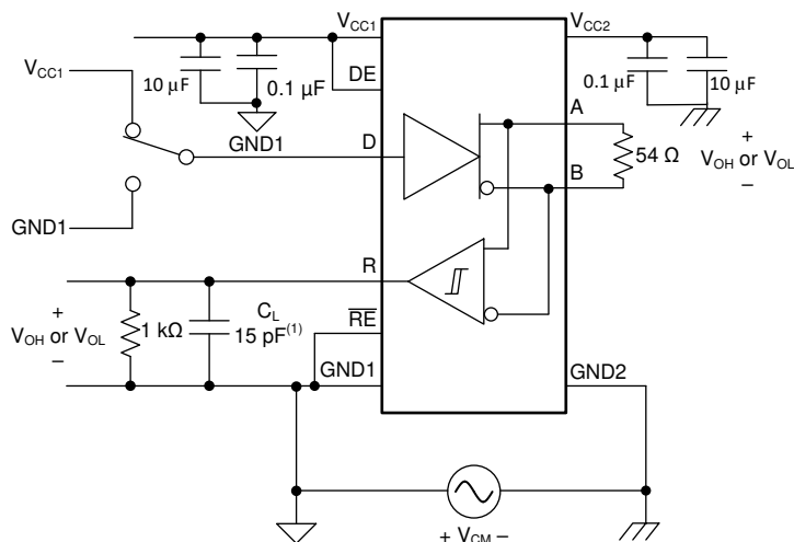
图 8-5. 共模瞬态抗扰度 (CMTI) — 半双工
