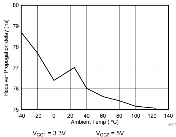
图 7-25. ISO143x 接收器传播延迟 (ns) 与温度 (C) 间的关系
