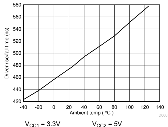
图 7-16. ISO141x 驱动器上升/下降时间 (ns) 与温度 (c) 间的关系
