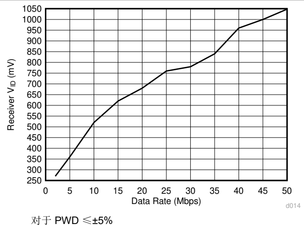
图 7-28. ISO145x 接收器 V_{ID} 与信令速率间的关系
