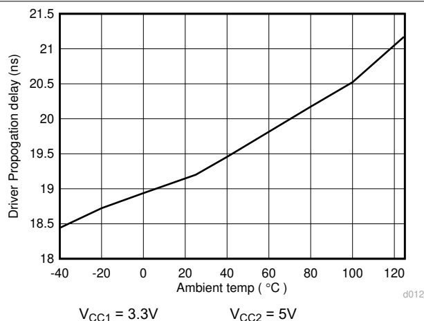
图 7-21. ISO145x 驱动器传播延迟 (ns) 与温度 (C) 间的关系
