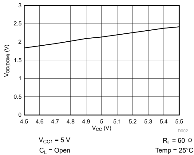
图 6-11. V_{\text{OD(DOM)}} Over V_{\text{CC}}
