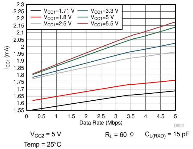
图 6-6. I_{CC1} vs Datarate
