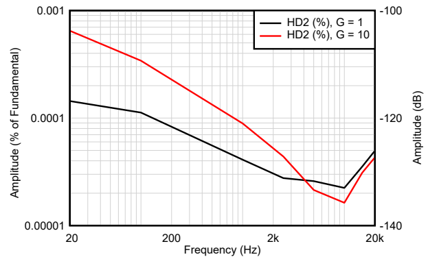
图 7-44. 第二谐波失真与频率间的关系
