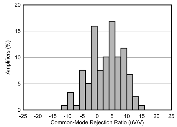
图 7-8. 典型 CMRR 分布 G = 1
