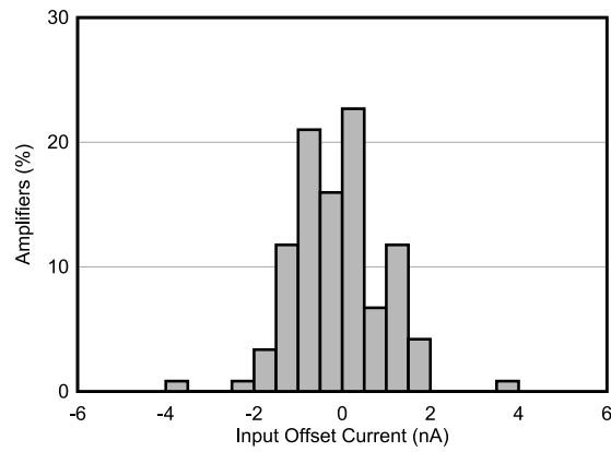
图 7-7. 输入失调电流的典型分布
