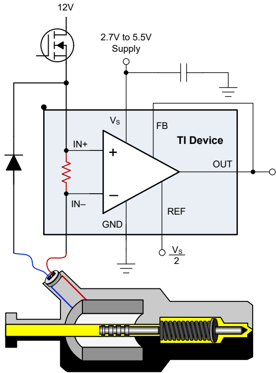
图 7-1. 螺线管驱动应用电路
