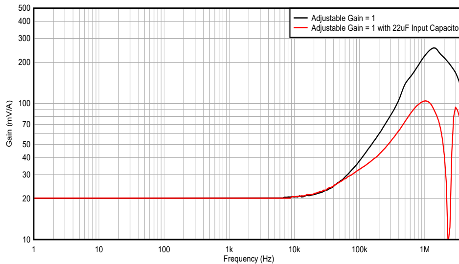
图 7-4. 添加 22μF 输入电容器之前和之后 INA791x 增益与频率间的关系
