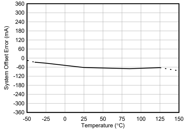
图 5-4. INA791B 输入失调电流与温度间的关系
