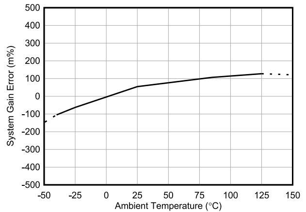
图 5-14. INA791B 增益误差与温度间的关系
