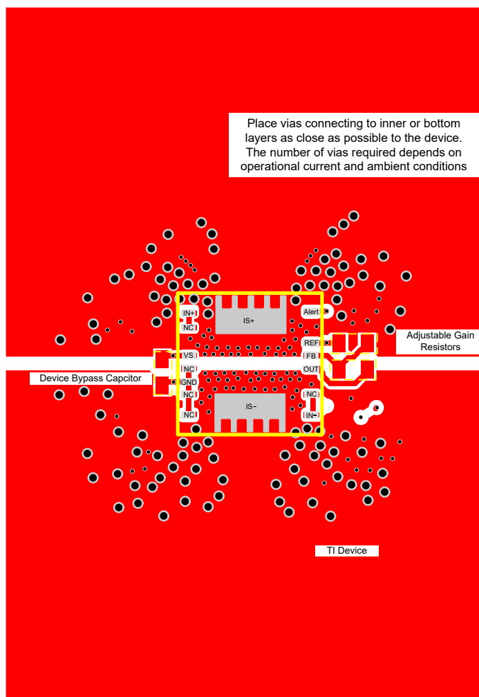
图 7-10. INA791x 布局示例
