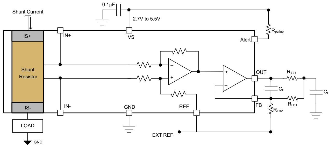
图 7-5. 具有 RISO 双反馈的 INA791x
