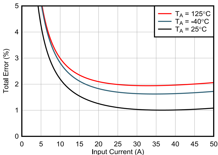
图 7-1. INA791A 总误差与输入电流间的关系
