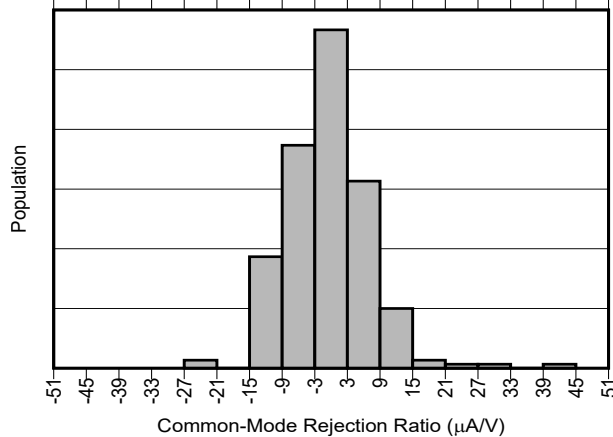
图 5-5. INA791A 共模抑制产生分布图
