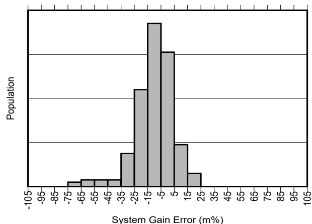
图 5-11. INA791A 增益误差产生分布图
