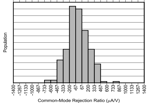
图 5-6. INA791B 共模抑制产生分布图
