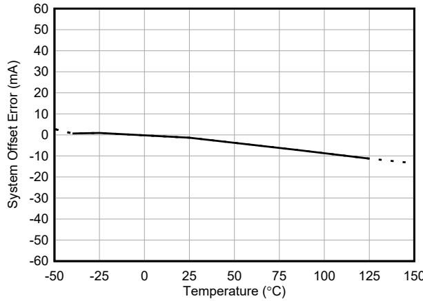
图 5-3. INA791A 输入失调电流与温度间的关系
