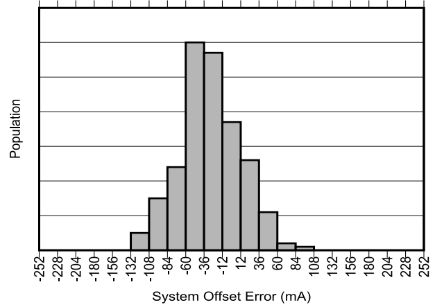
图 5-2. INA791B 输入失调电流产生分布图
