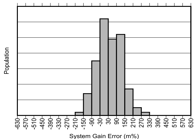
图 5-12. INA791B 增益误差产生分布图
