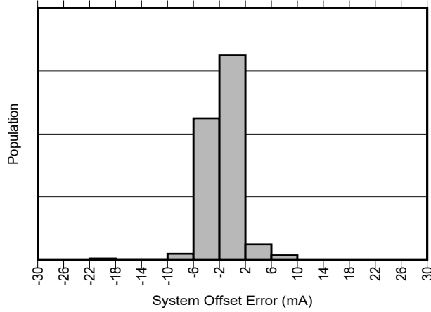
图 5-1. INA791A 输入失调电流产生分布图
