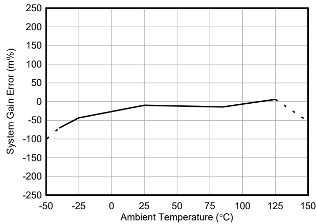
图 5-13. INA791A 增益误差与温度间的关系
