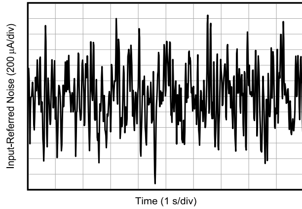
图 5-27. 以输入为基准的 0.1Hz 至 10Hz 电流噪声
