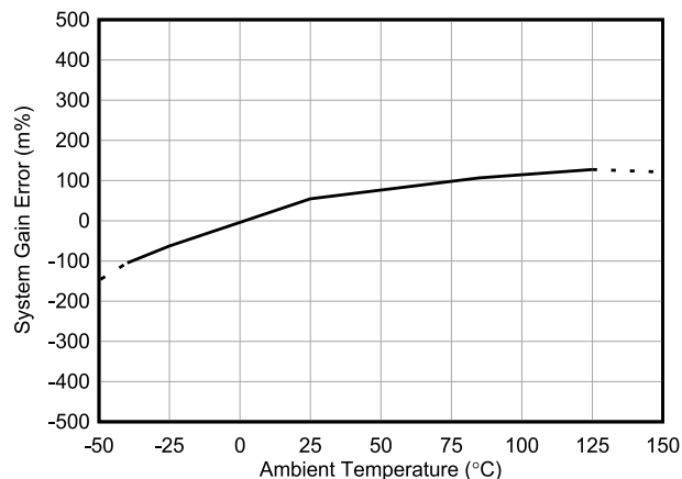
图 5-8. INA790B 增益误差与温度间的关系
