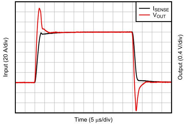
图 5-28. 系统电流阶跃响应
