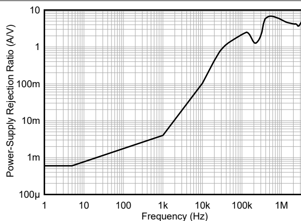
图 5-12. 电源抑制比与频率间的关系
