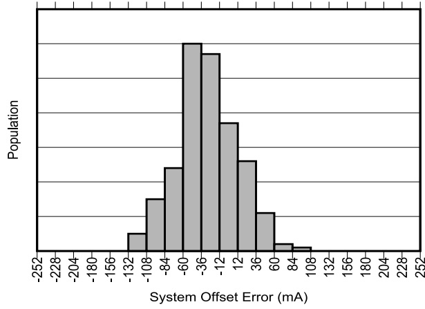
图 5-1. INA790B 输入失调电流产生分布图
