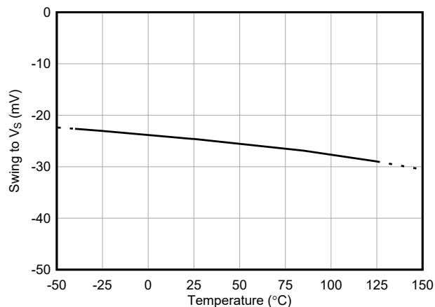
图 5-17. 输出电压摆幅高位与温度间的关系
