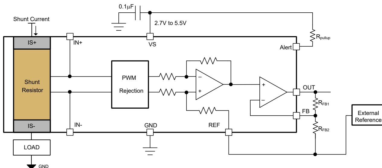
图 6-10. 热警报功能
