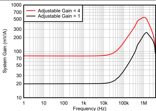
图 5-11. 系统增益与频率间的关系
