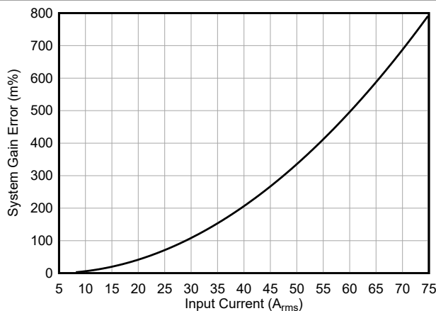
图 5-9. INA790B 系统增益误差与输入电流间的关系
