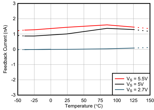
图 5-25. 反馈电流与温度间的关系
