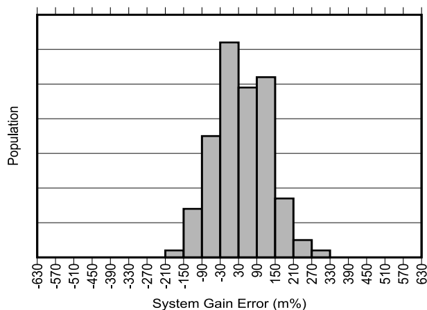
图 5-7. INA790B 增益误差产生分布图
