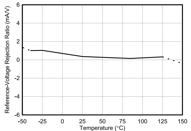
图 5-6. 基准电压抑制比与温度间的关系
