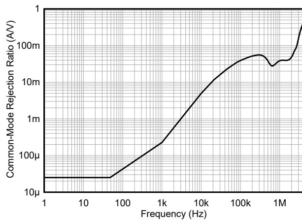
图 5-13. 共模抑制比与频率间的关系
