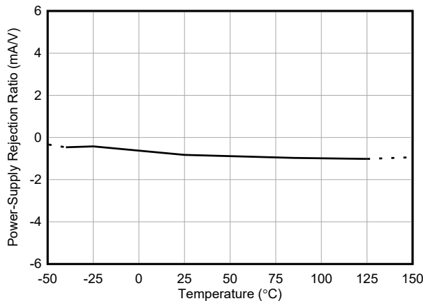
图 5-5. 电源抑制比与温度间的关系
