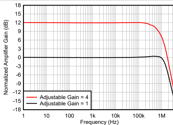
图 5-10. 电流检测放大器增益与频率间的关系
