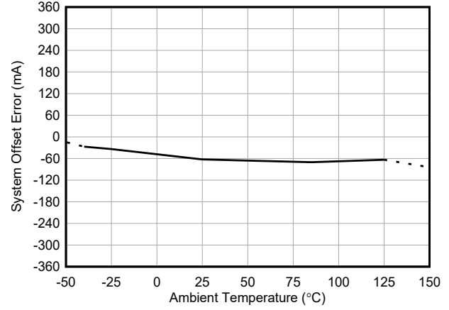
图 5-2. INA790B 输入失调电流与温度间的关系
