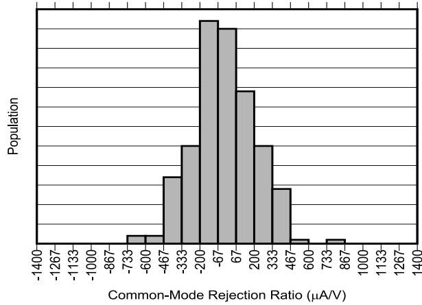
图 5-3. INA790B 共模抑制产生分布图
