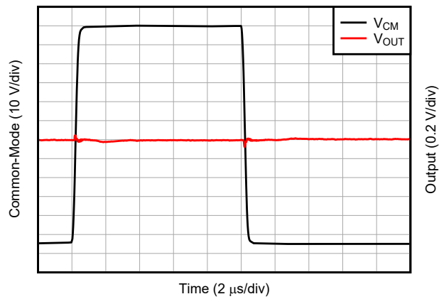
图 5-29. -4V 至 110V 共模阶跃瞬态响应
