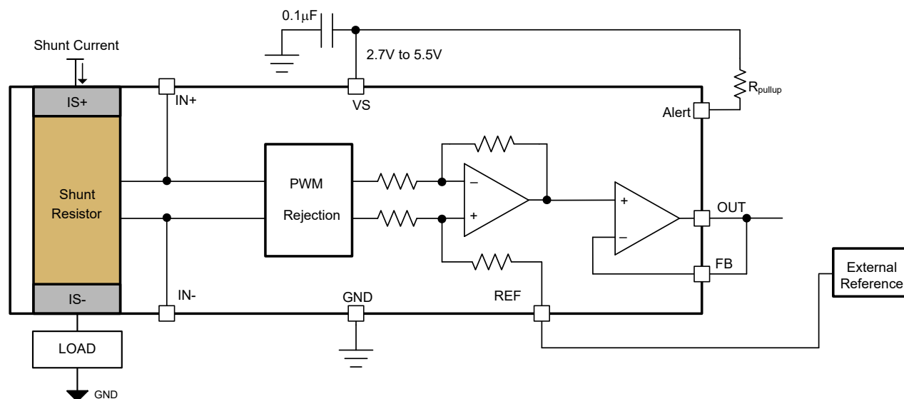
图 6-9. 可调单位增益设置
