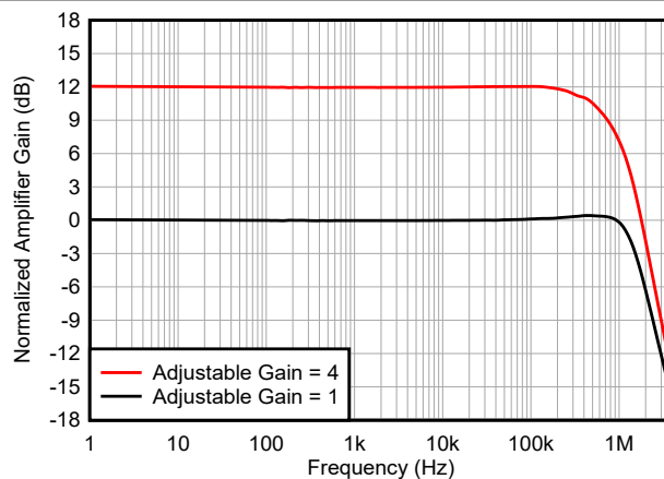
图 5-10. 电流检测放大器增益与频率间的关系
