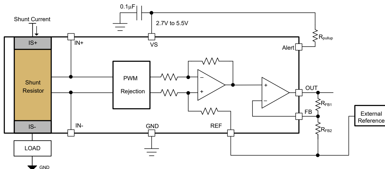
图 6-10. 热警报功能
