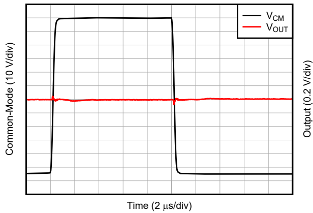
图 5-29. 共模瞬态响应
