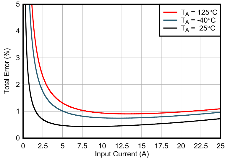
图 7-1. INA750A 总误差与输入电流间的关系
