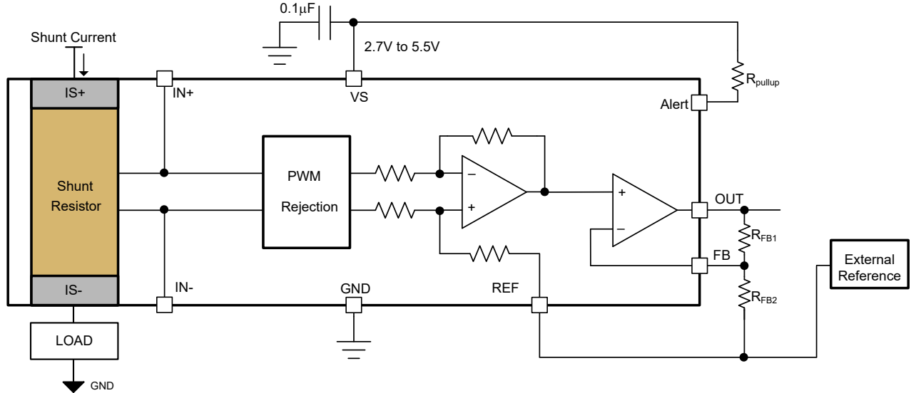
图 6-5. 调节输出
