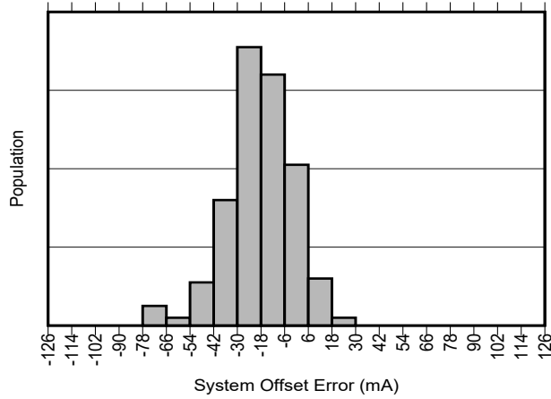
图 5-1. INA750 B 输入失调电流产生分布图
