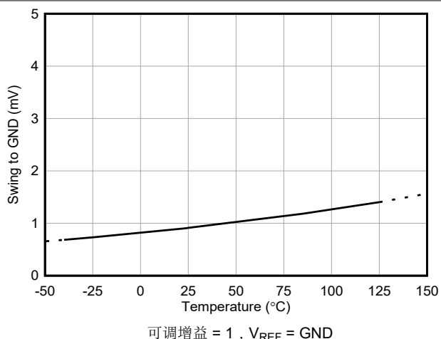
图 5-18. 输出电压摆幅低位与温度间的关系
