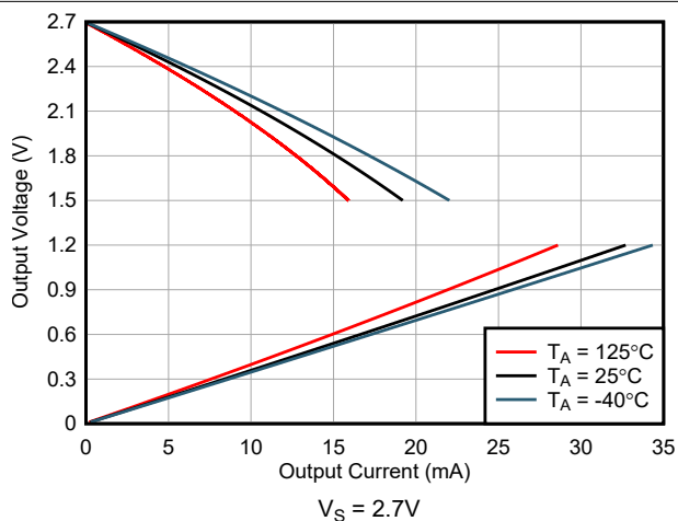
图 5-14. 输出电压摆幅与输出电流间的关系
