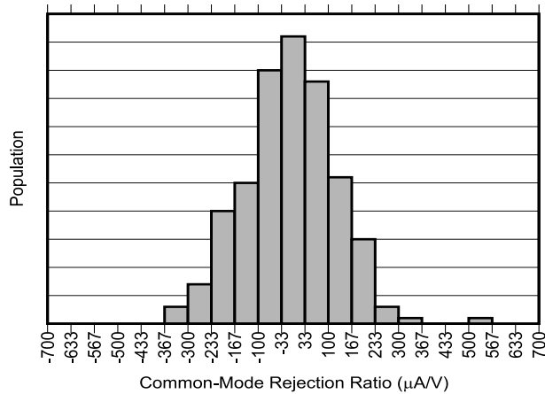
图 5-3. INA750 B 共模抑制产生分布图
