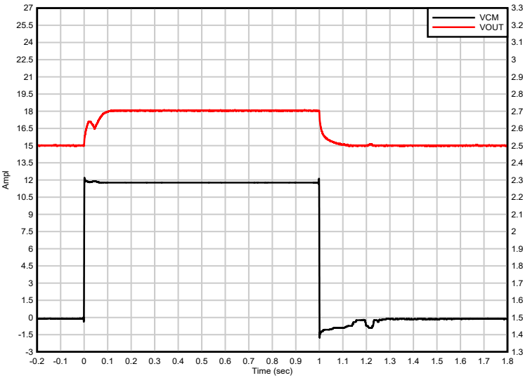
图 7-9. 螺线管驱动电流检测输入和输出信号
