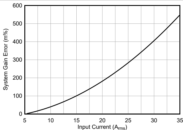
图 5-9. INA750 B 系统增益误差与输入电流间的关系
