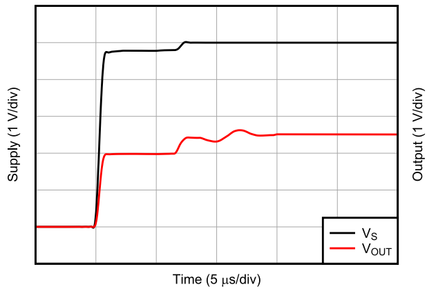
图 5-28. 放大器阶跃响应
