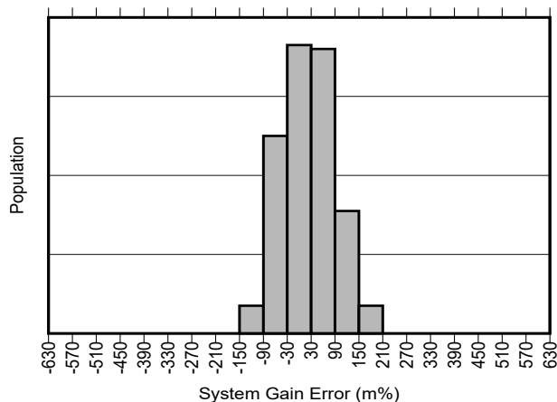
图 5-7. INA750 B 增益误差产生分布图
