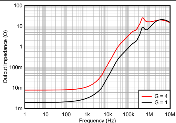
图 5-16. 输出阻抗与频率间的关系
