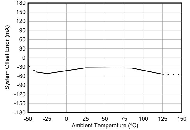
图 5-2. INA750 B 输入失调电流与温度间的关系
