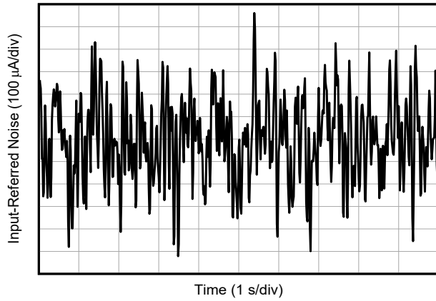
图 5-27. 0.1Hz 至 10Hz 电压噪声 (以输入为基准)
