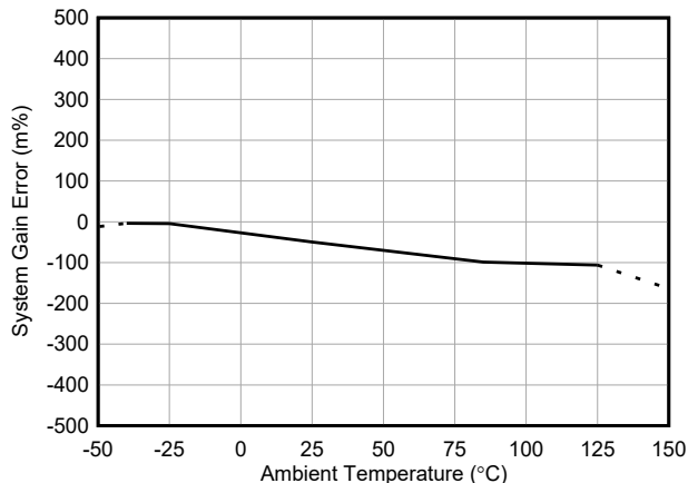
图 5-8. INA750 B 增益误差与温度间的关系
