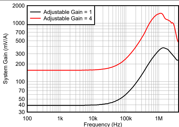
图 5-11. 系统增益与频率间的关系
