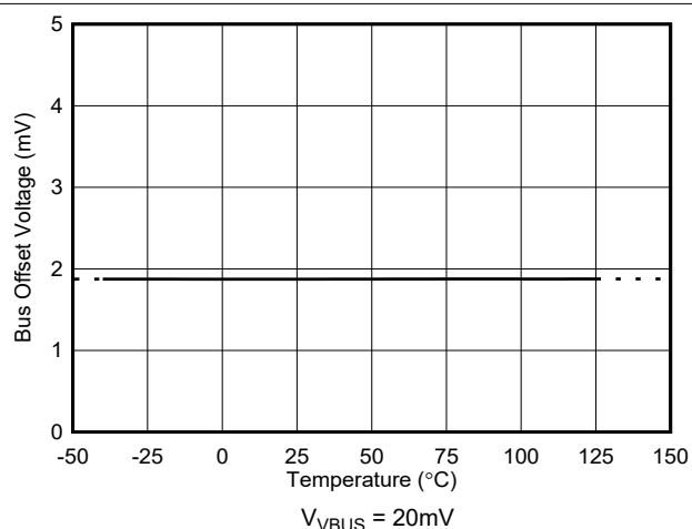
图 5-10. 总线输入失调电压与温度间的关系 V_{VBUS} = 20\text{mV}
