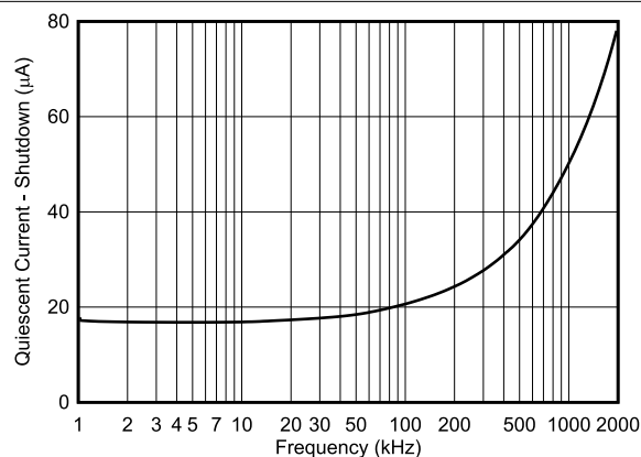
图 5-21. 关断 I_Q 与时钟频率间的关系
