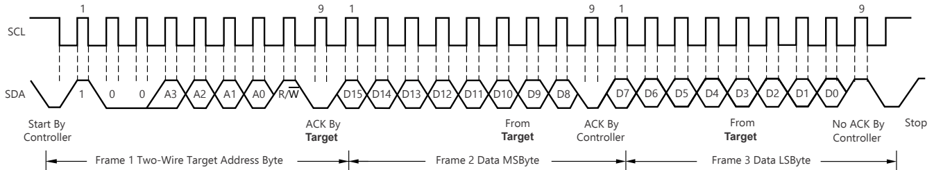
图 6-12. 写入字格式的时序图
