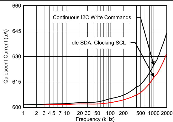
图 5-20. 工作 I_Q 与时钟频率间的关系
