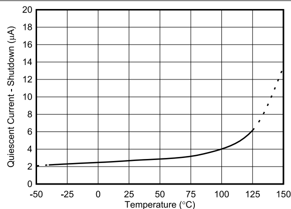
图 5-19. 关断 I_Q 与温度间的关系
