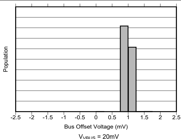
图 5-9. 总线输入失调电压产生分布图 V_{VBUS} = 20\text{mV}
