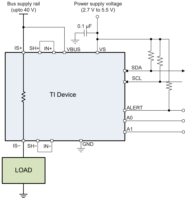
图 7-2. INA745x 高侧感测应用图
