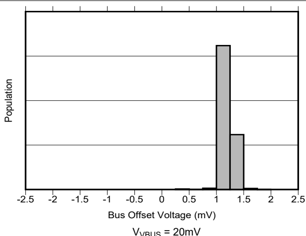
图 5-9. 总线输入失调电压产生分布图
