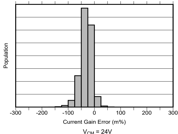
图 5-6. 电流增益误差产生分布图
