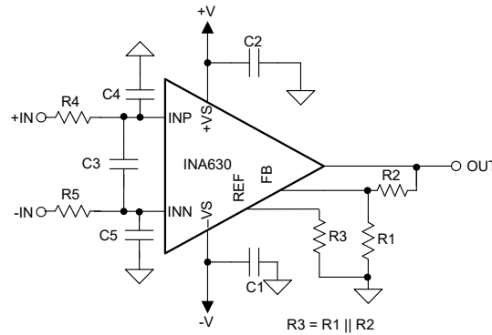
图 8-5. 示例原理图
