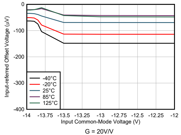
图 6-16. 失调电压与负共模电压间的关系 G = 20\text{V/V}
