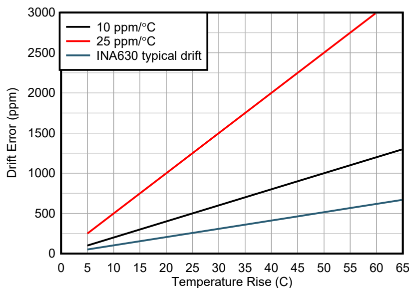
图 8-4. 典型误差漂移 (ppm) 与温度上升 ( ^\circ\text{C} ) 的关系
