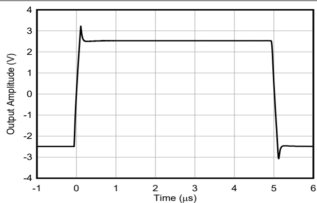
图 6-28. 大信号阶跃响应
