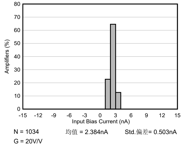
图 6-2. 正输入偏置电流的典型分布, T_A = 25^\circ\text{C}
