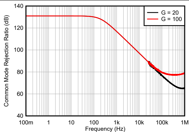
图 6-5. CMRR 与频率间的关系 (RTI)
