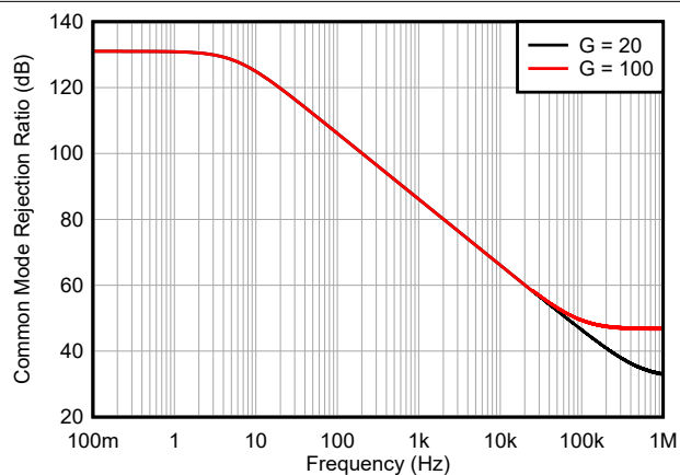
图 6-6. CMRR 与频率间的关系 (RTI, 1kΩ 源不平衡)
