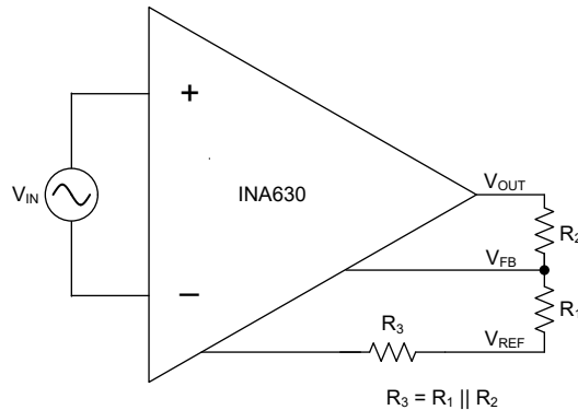
图 7-5. FB 引脚偏置电流补偿
