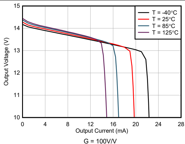
图 6-18. 正输出电压摆幅与输出电流间的关系
