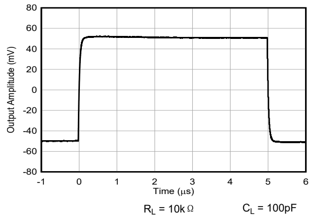
图 6-26. 小信号响应, G = 20\text{V/V}
