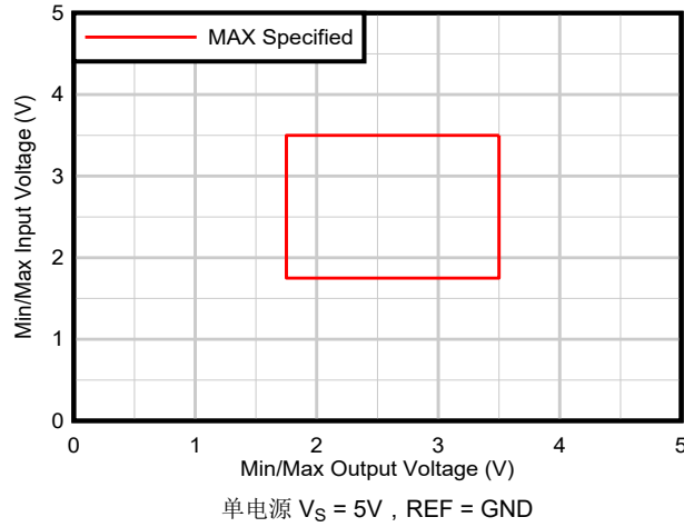
图 6-21. 输入电压 与输出电压间的关系 (双电源 V_S = 5\text{V} )
