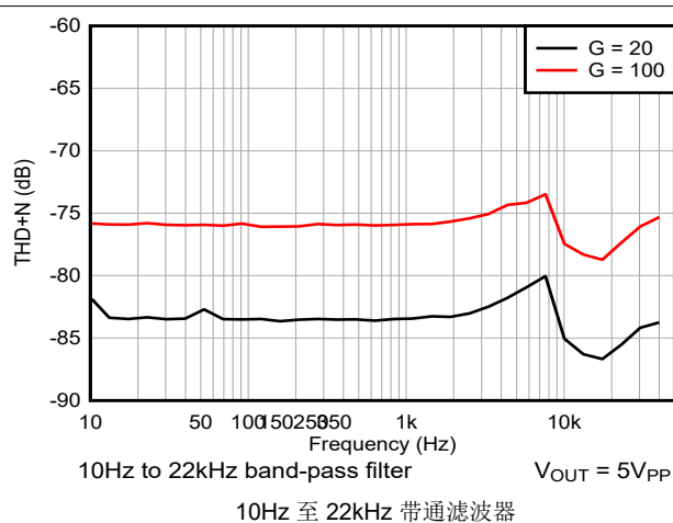
图 6-31. 总谐波失真与频率间的关系, 10Hz 至 22kHz
