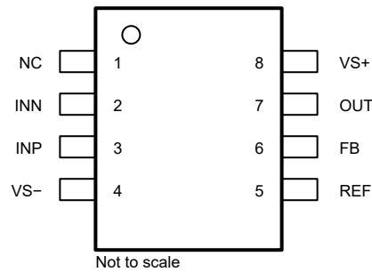
图 5-1. DDF 封装，8 引脚 SOT-23 ( 顶视图 )
