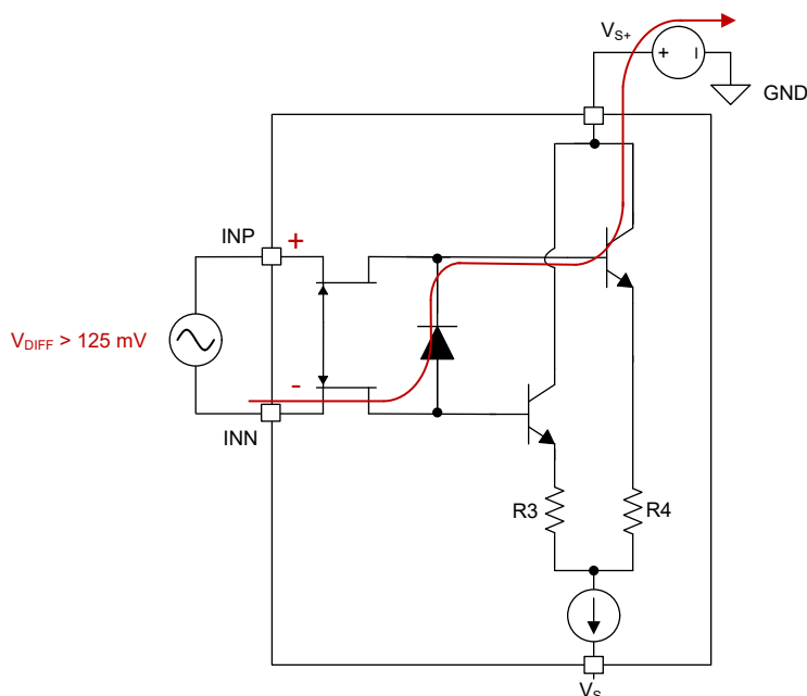
图 7-6. 大差分输入电压条件下的输入电流路径
