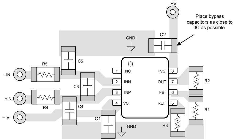
图 8-6. 相关 PCB 布局
