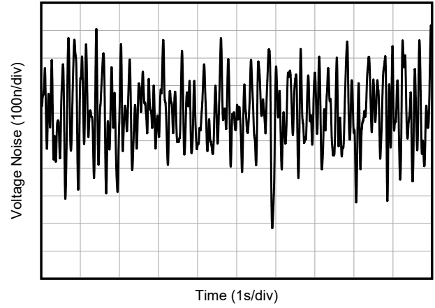
图 6-12. 0.1Hz 至 10Hz RTI 电压噪声, G = 100\text{V/V}
