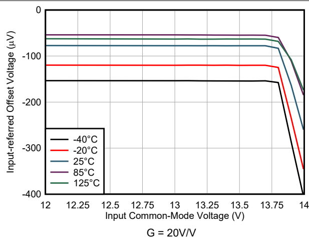
图 6-17. 失调电压与正共模电压间的关系
