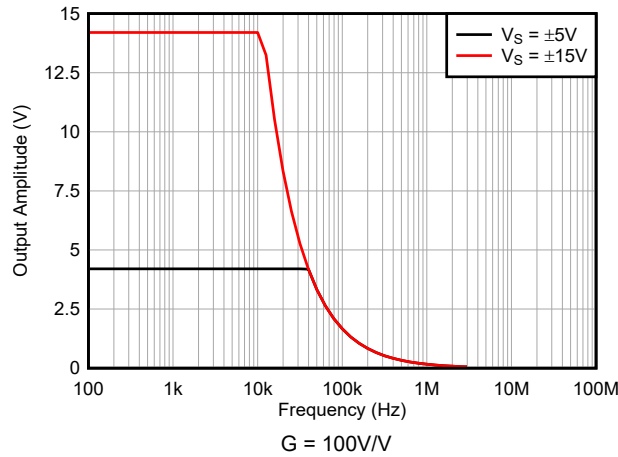
图 6-23. 大信号频率响应, G = 100\text{V/V}
