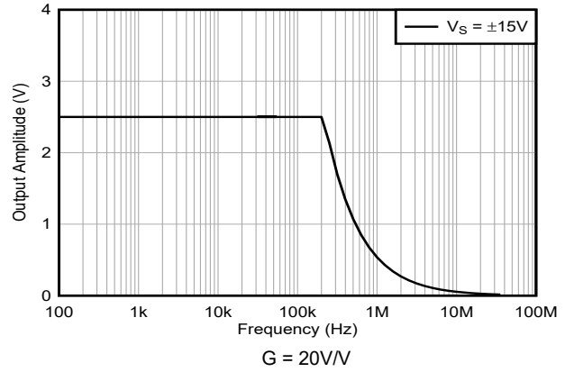
图 6-22. 大信号频率响应, G = 20\text{V/V}
