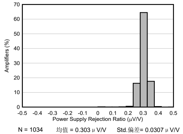
图 6-4. 典型 PSRR 分布, G = 20\text{V/V}
