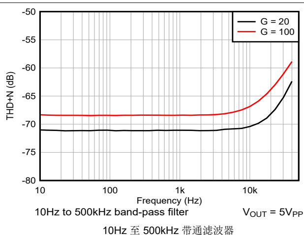
图 6-32. 总谐波失真与频率间的关系, 10Hz 至 500kHz
