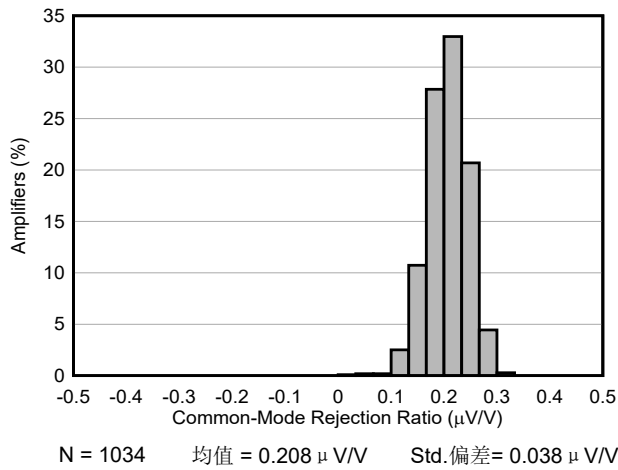
图 6-3. 典型 CMRR 分布, G = 20\text{V/V}
