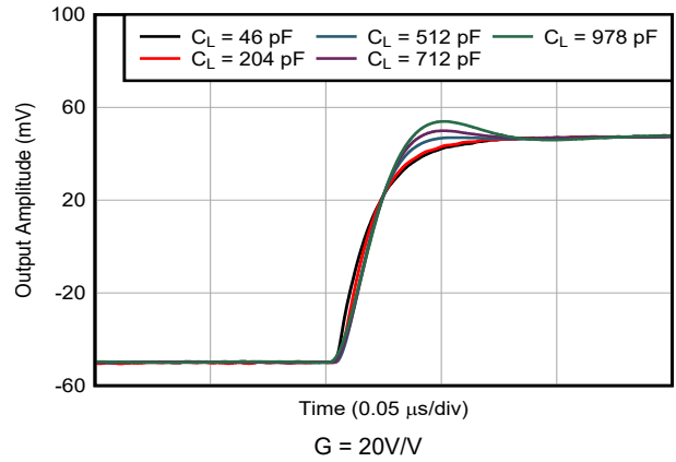
图 6-24. 过冲与容性负载间的关系, 上升
