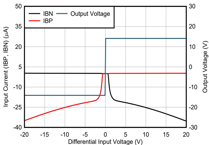
图 7-7. 输入电流 (IBP、IBN) 与差分输入电压的关系
