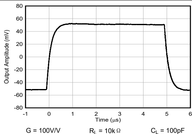
图 6-27. 小信号响应, G = 100\text{V/V}
