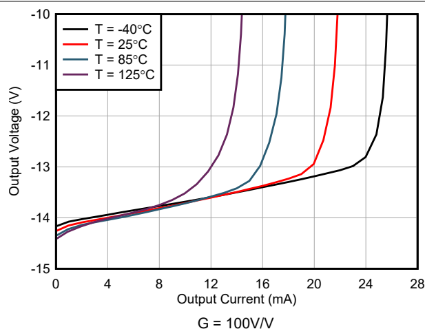
图 6-19. 负输出电压摆幅与输出电流间的关系
