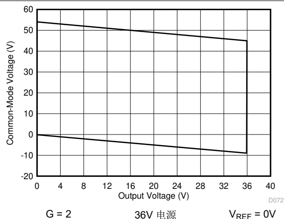
图 7-72. 输入共模电压与输出电压间的关系
