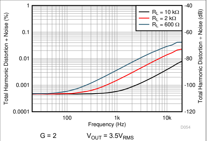
图 7-54. THD+N 与频率间的关系
