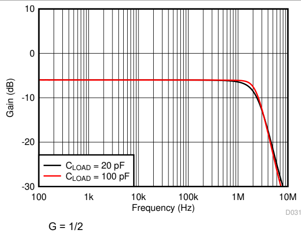
图 7-31. 闭环增益与频率间的关系
