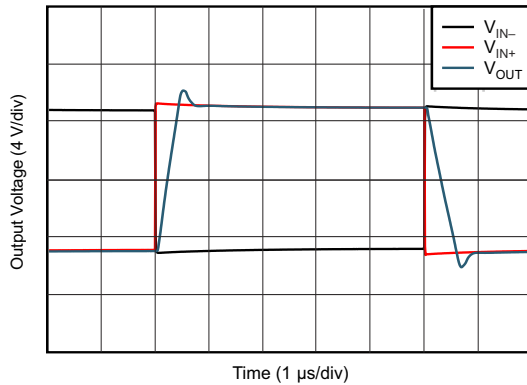
图 7-43. 建立时间
