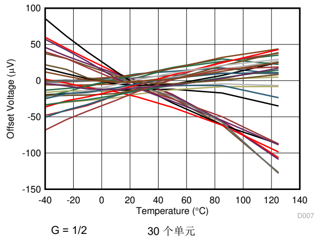
图 7-7. 输出失调电压与温度间的关系
