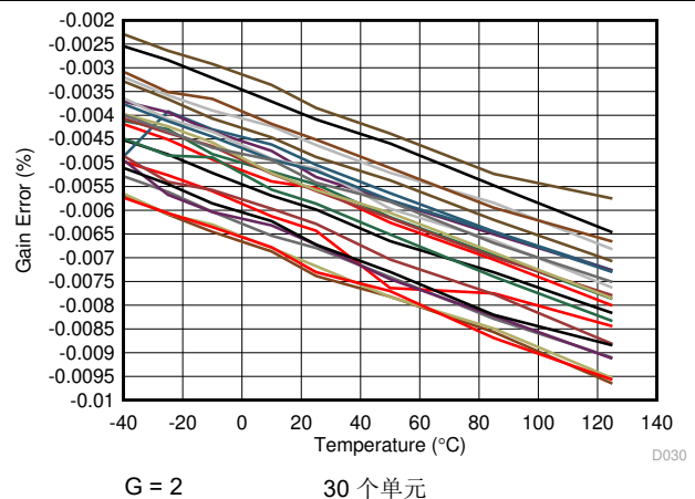
图 7-30. 增益误差与温度间的关系
