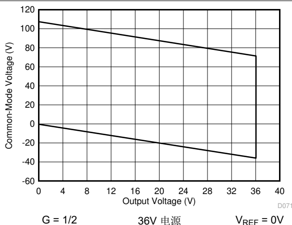
图 7-71. 输入共模电压与输出电压间的关系
