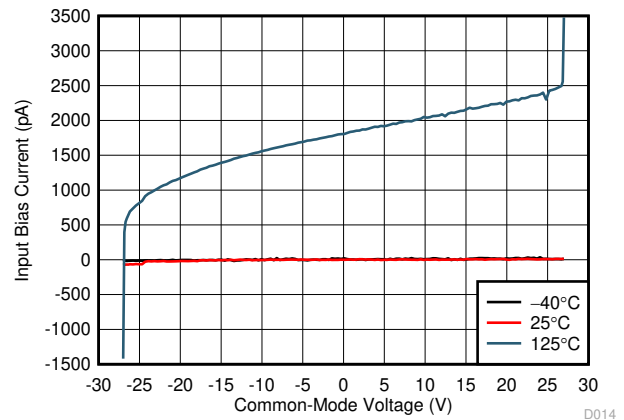
图 7-14. 输入偏置电流与共模电压间的关系
