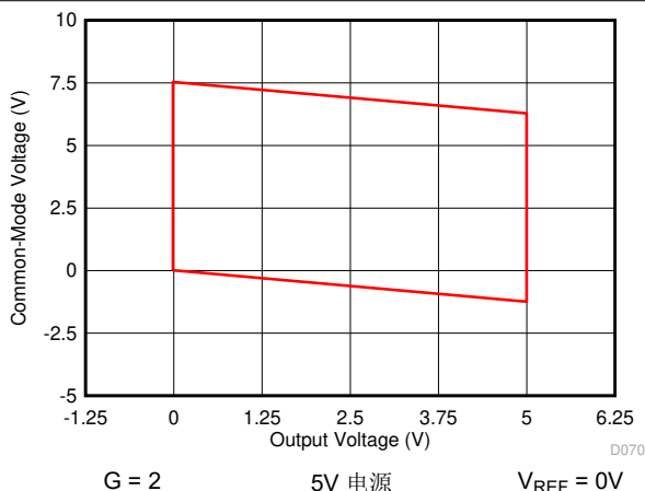
图 7-70. 输入共模电压与输出电压间的关系
