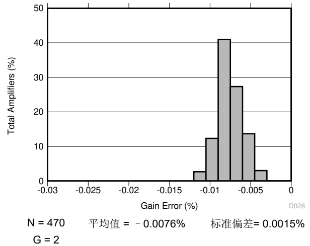
图 7-28. 增益误差的典型分布
