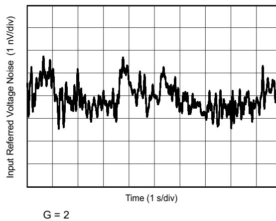
图 7-36. 0.1Hz 至 10Hz RTI 电压噪声
