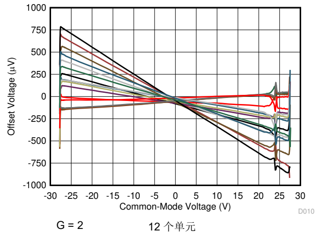
图 7-10. 失调电压与共模电压间的关系
