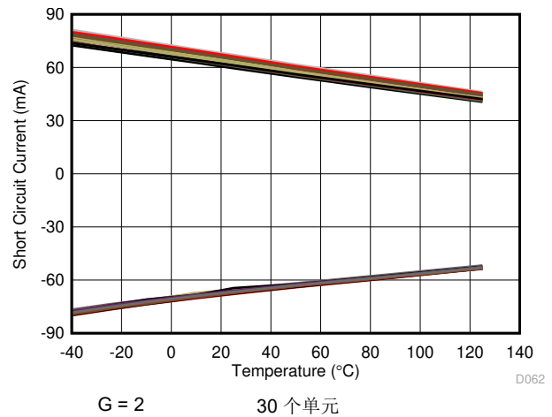
图 7-62. 短路电流与温度间的关系
