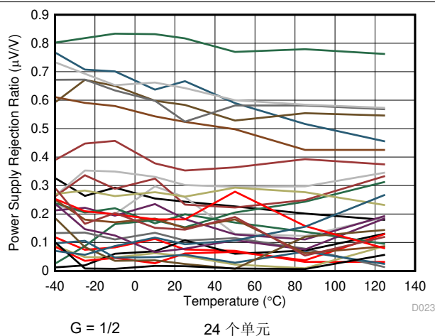
图 7-23. PSRR 与温度间的关系
