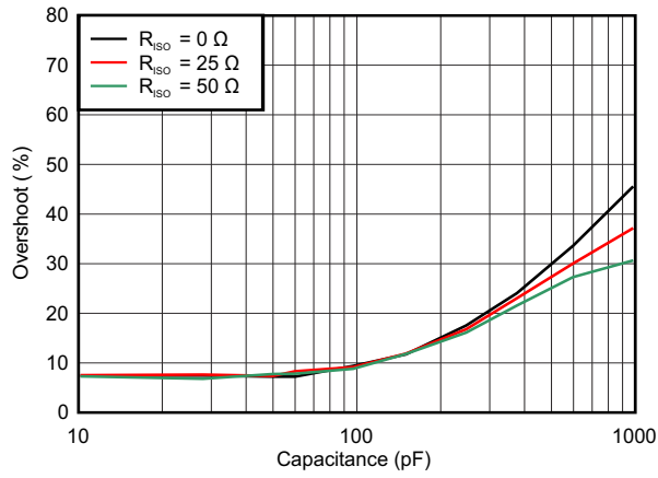
图 7-49. 小信号过冲与容性负载间的关系
