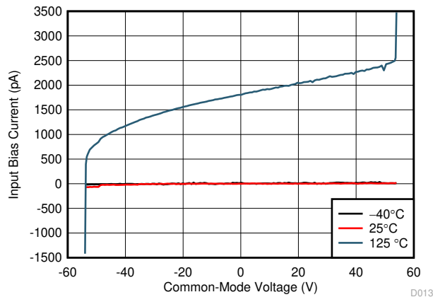
图 7-13. 输入偏置电流与共模电压间的关系
