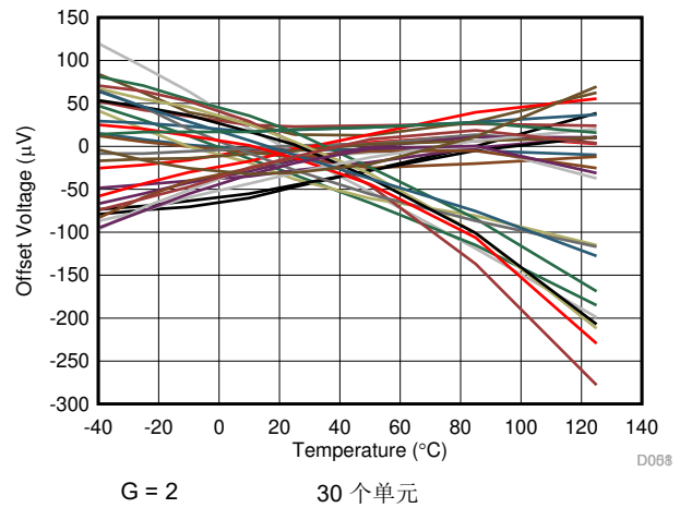
图 7-8. 输出失调电压与温度间的关系
