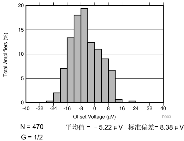
图 7-3. 失调电压的典型分布 (RTO)
