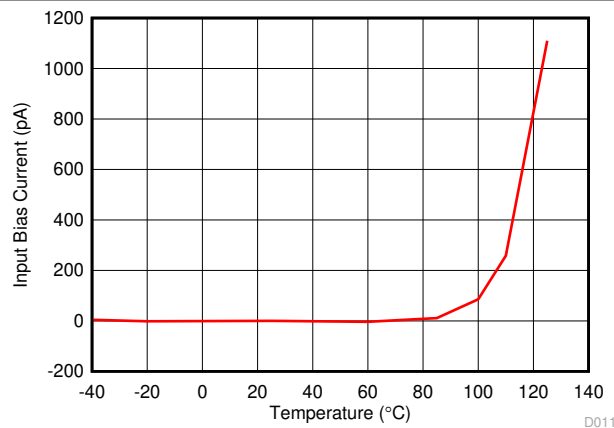
图 7-11. 输入偏置电流与温度间的关系
