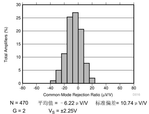
图 7-16. 典型 CMRR 分布
