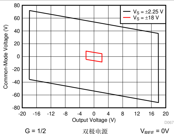
图 7-67. 输入共模电压与输出电压间的关系
