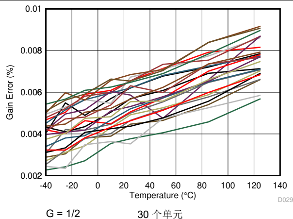
图 7-29. 增益误差与温度间的关系
