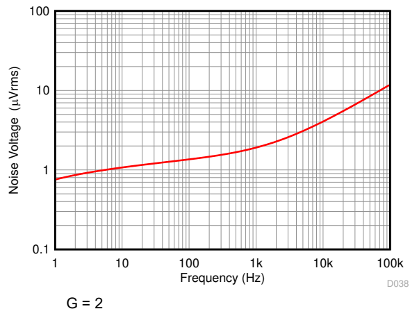
图 7-38. 集成输出电压噪声与噪声带宽间的关系
