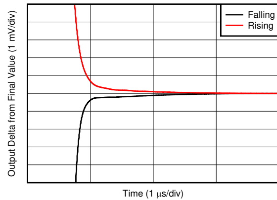
图 7-44. 建立时间
