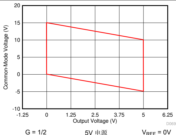
图 7-69. 输入共模电压与输出电压间的关系
