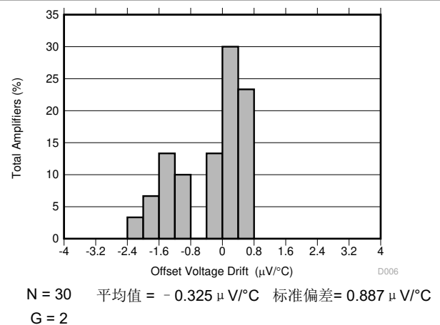
图 7-6. 失调电压漂移的典型分布 (RTO)
