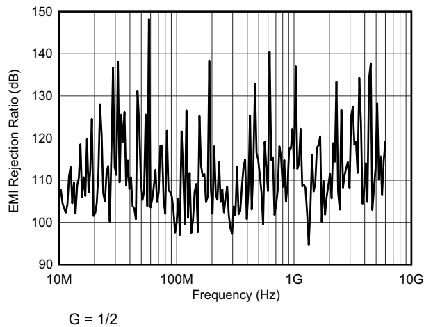
图 7-63. 差模 EMI 抑制比
