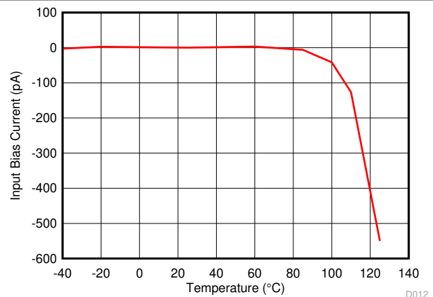
图 7-12. 输入失调电流与温度间的关系
