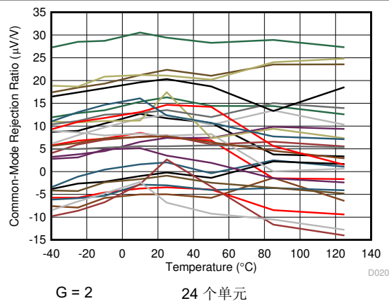
图 7-20. CMRR 与温度间的关系
