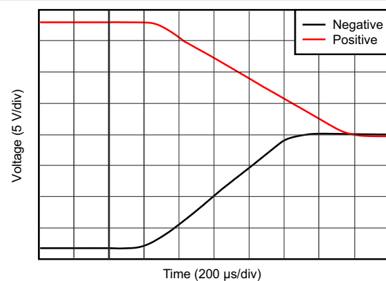
图 7-46. 大信号阶跃响应
