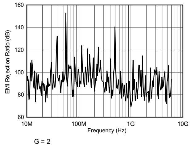
图 7-64. 差模 EMI 抑制比
