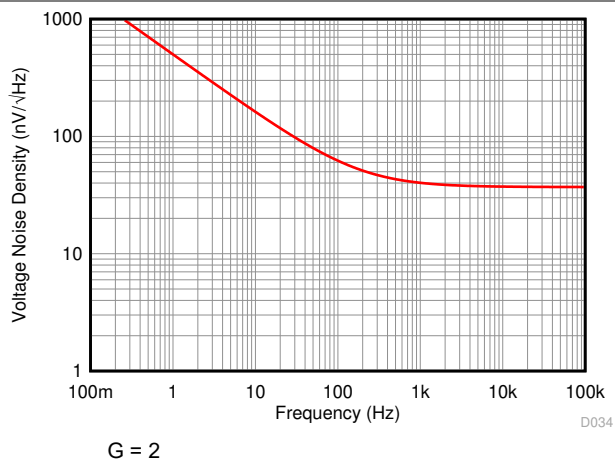
图 7-34. 电压噪声频谱密度与频率间的关系 (RTI)
