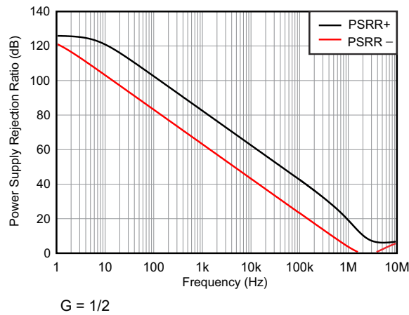
图 7-25. PSRR 与频率间的关系 (RTI)
