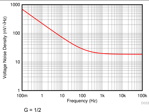
图 7-33. 电压噪声频谱密度与频率间的关系 (RTI)
