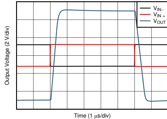
图 7-44. 建立时间
