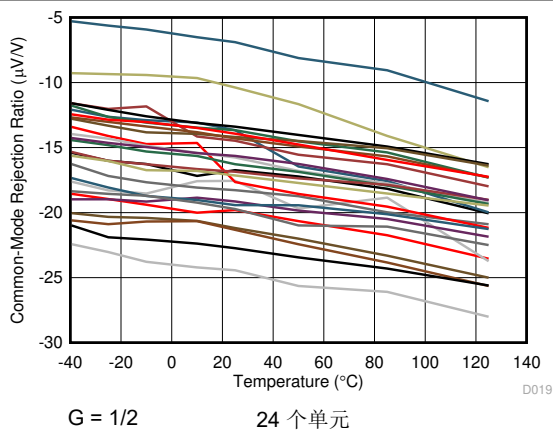
图 7-19. CMRR 与温度间的关系
