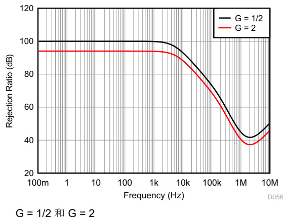
图 7-21. 共模抑制比与频率之间的关系, 以输入为基准
