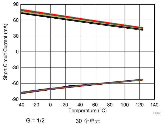
图 7-61. 短路电流与温度间的关系
