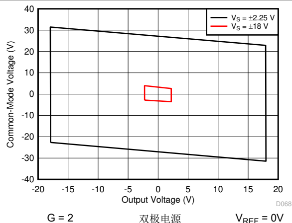
图 7-68. 输入共模电压与输出电压间的关系
