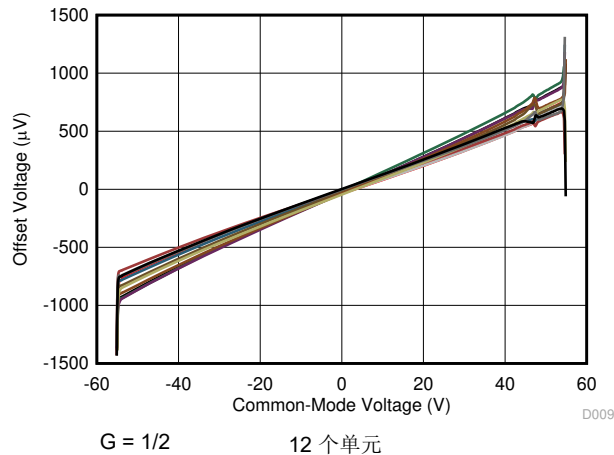
图 7-9. 失调电压与共模电压间的关系
