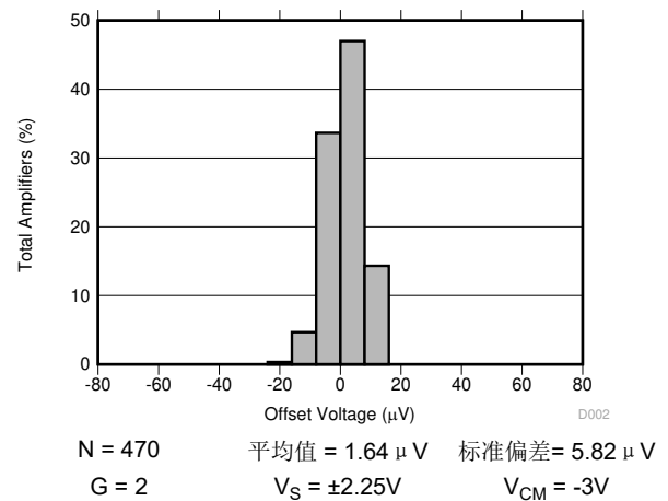
图 7-2. 失调电压的典型分布 (RTO)
