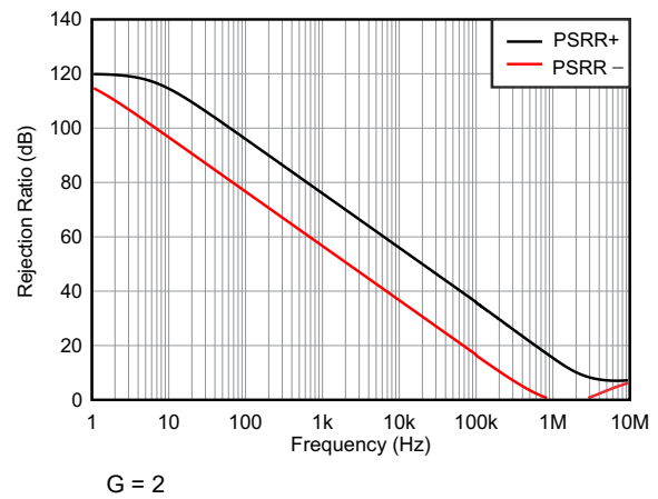
图 7-26. PSRR 与频率间的关系 (RTI)
