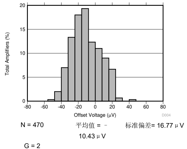
图 7-4. 失调电压的典型分布 (RTO)
