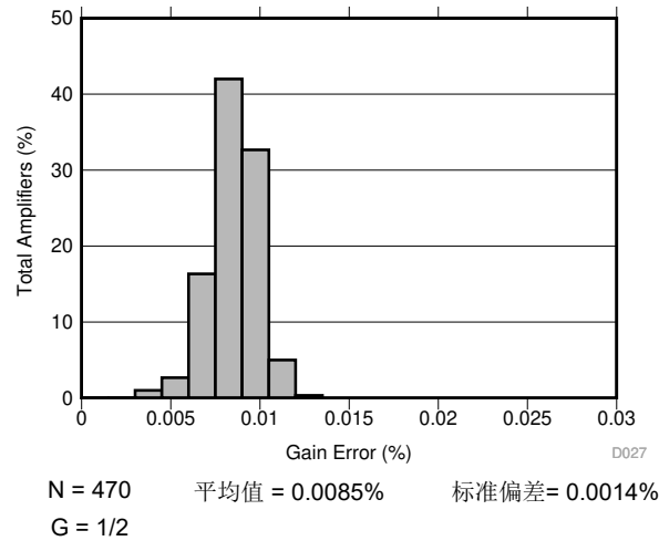
图 7-27. 增益误差的典型分布
