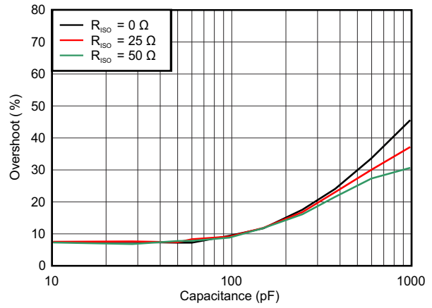
图 7-50. 小信号过冲与容性负载间的关系
