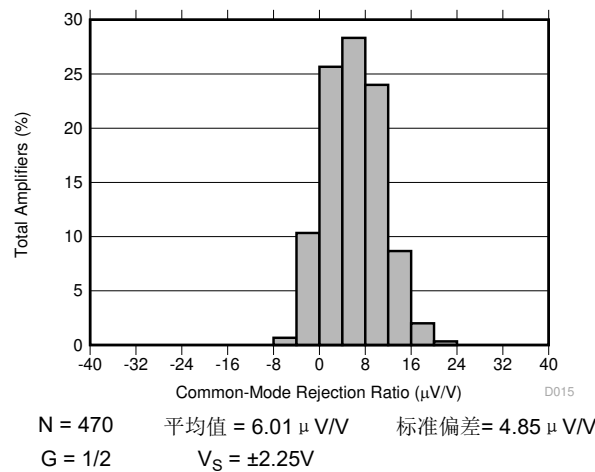
图 7-15. 典型 CMRR 分布
