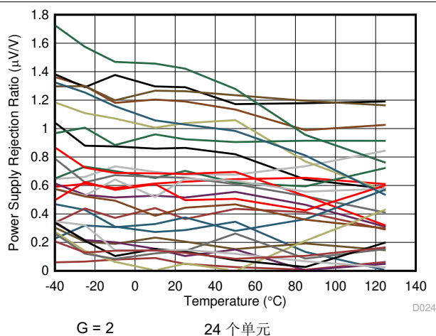
图 7-24. PSRR 与温度间的关系
