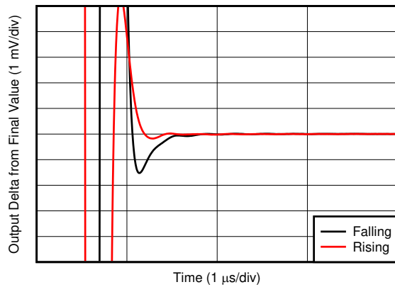
图 7-43. 建立时间
