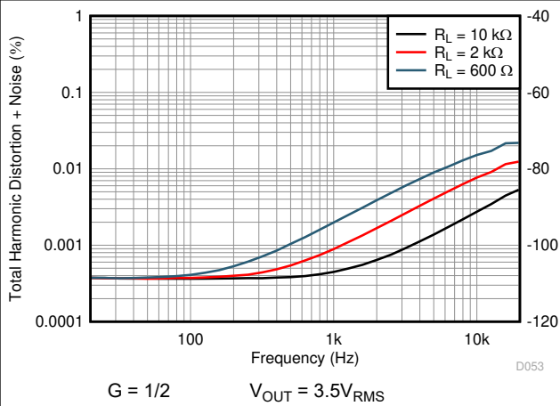
图 7-53. THD+N 与频率间的关系
