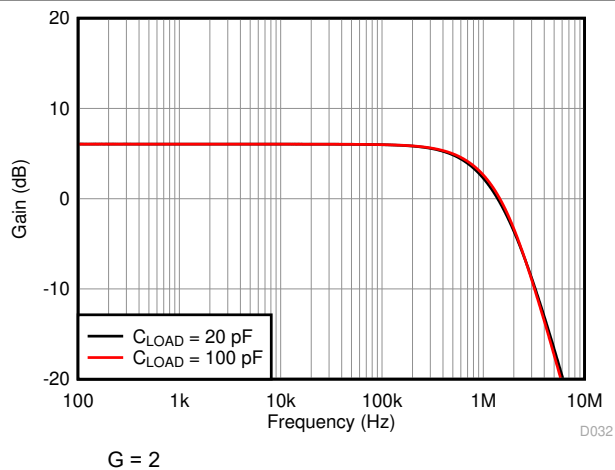
图 7-32. 闭环增益与频率间的关系
