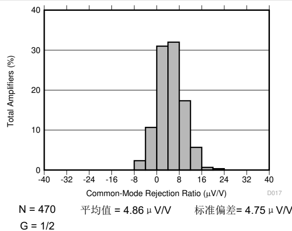
图 7-17. 典型 CMRR 分布
