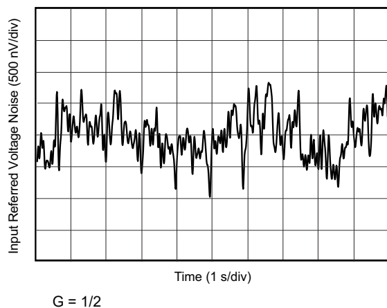
图 7-35. 0.1Hz 至 10Hz RTI 电压噪声
