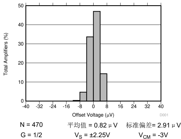
图 7-1. 失调电压的典型分布 (RTO)
