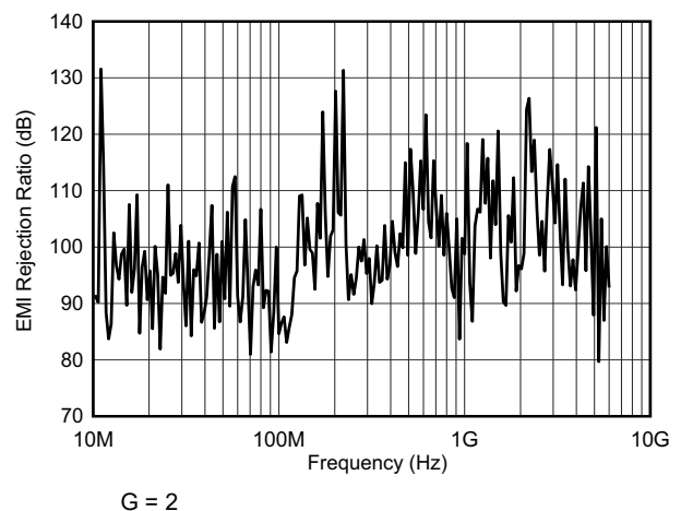
图 7-66. 共模 EMI 抑制比
