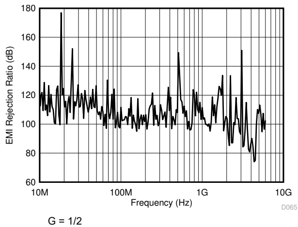
图 7-65. 共模 EMI 抑制比
