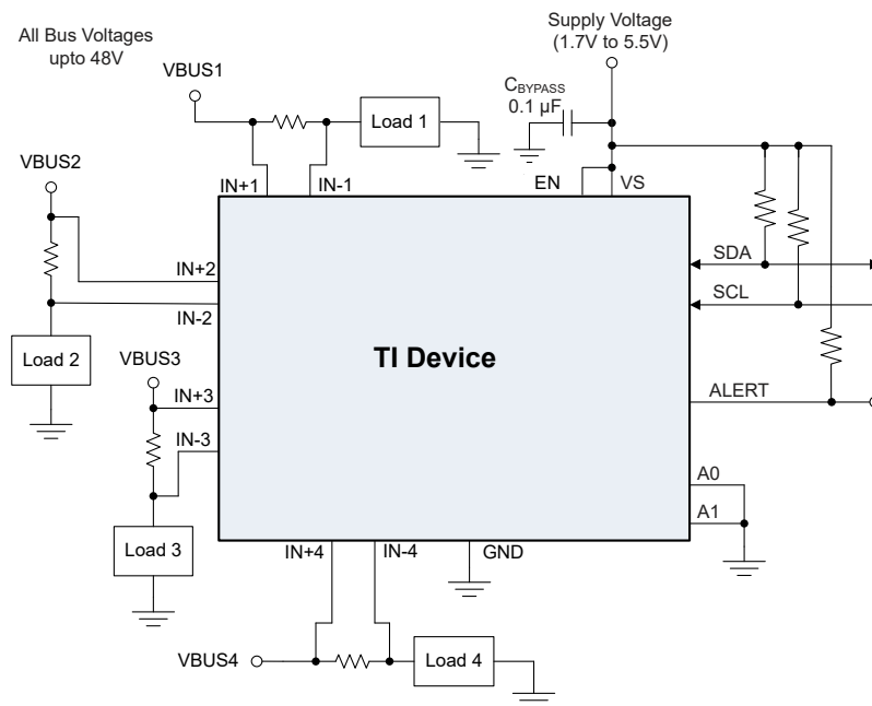
图 8-2. 典型的高侧检测电路配置，INA4235
