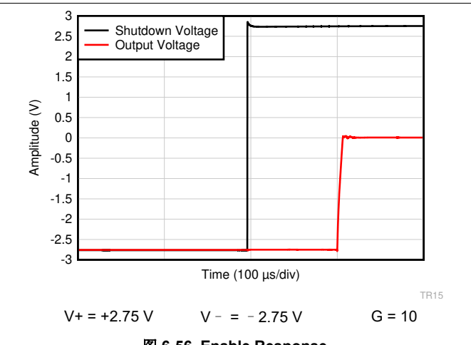
图 6-56. Enable Response
