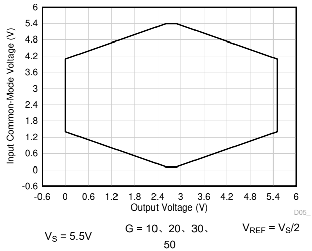
图 8-2. 输入共模电压与输出电压间的关系
