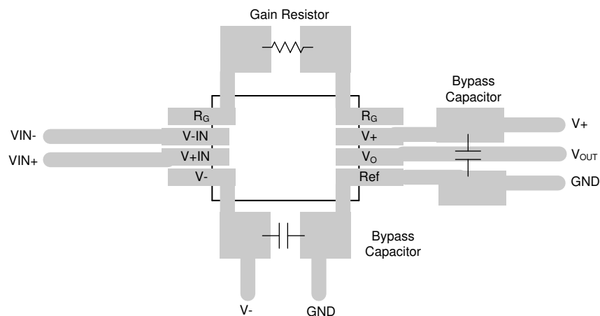
图 8-9. Layout Example
