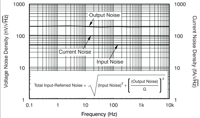
图 6-8. Spectral Noise Density
