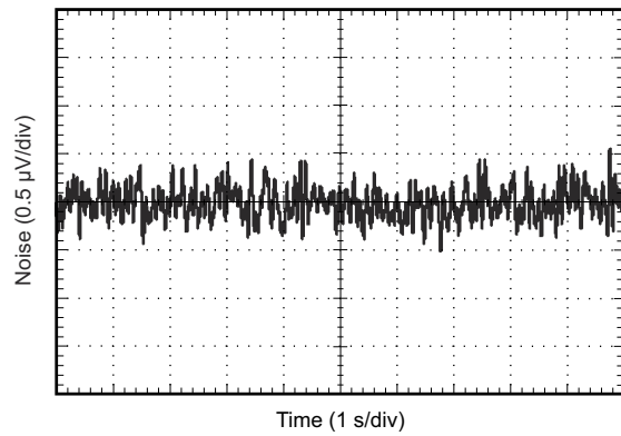
图 6-7. 0.1-Hz to 10-Hz Noise
