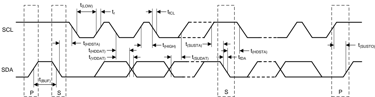
图 31. Bus Timing
