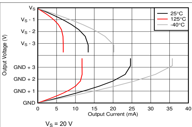
图 6-20. 输出电压与输出电流间的关系
