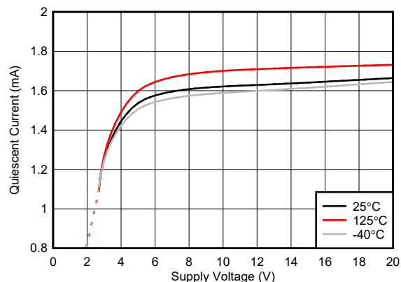
图 6-28. 静态电流与电源电压间的关系
