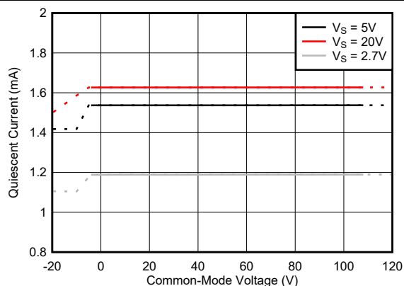
图 6-29. 静态电流与共模电压间的关系
