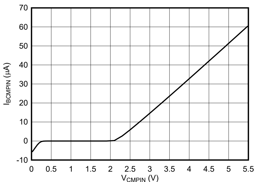
图 7-3. 比较器 I_{\text{BCMPIN}} 与 V_{\text{CMPIN}} 关系图
