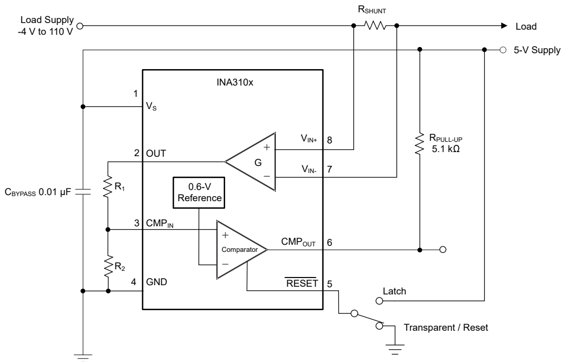
图 7-4. INA310x-Q1 基本连接
