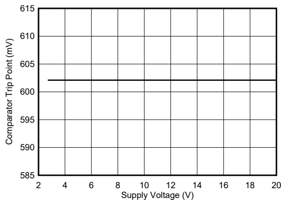
图 6-35. 比较器跳闸点与电源电压关系图
