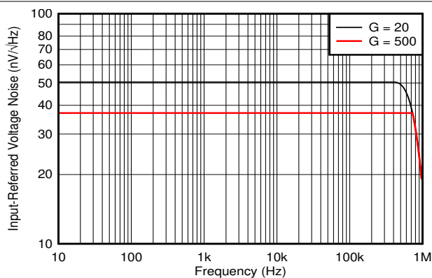
图 6-24. 输入参考噪声与频率间的关系
