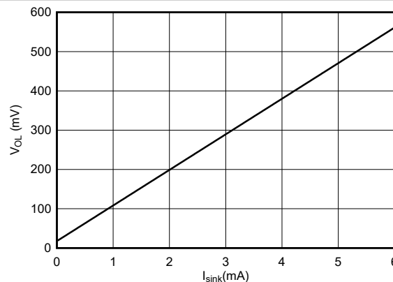
图 6-34. 比较器 V_{OL} 与 I_{SINK} 关系图
