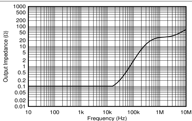
图 6-21. 输出阻抗与频率间的关系
