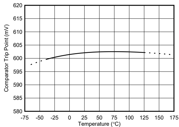
图 6-36. 比较器跳闸点与温度关系图
