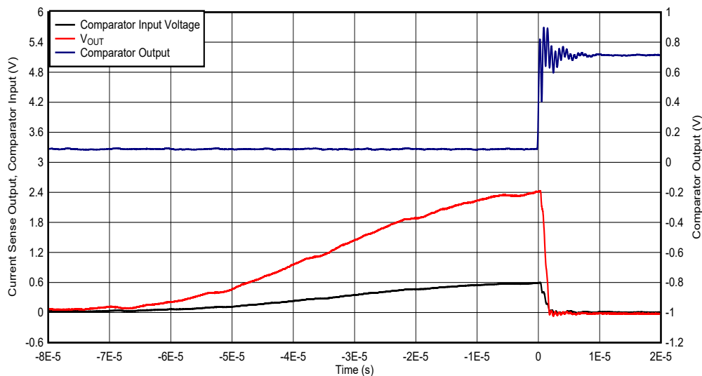
图 8-4. 低侧开关过流关断响应
