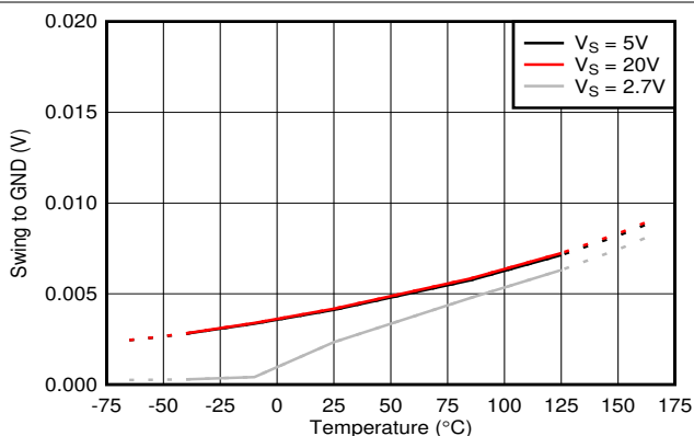
图 6-23. 相对于 GND 的摆幅与温度间的关系
