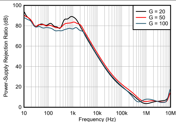
图 5-10. 电源抑制比与频率间的关系
