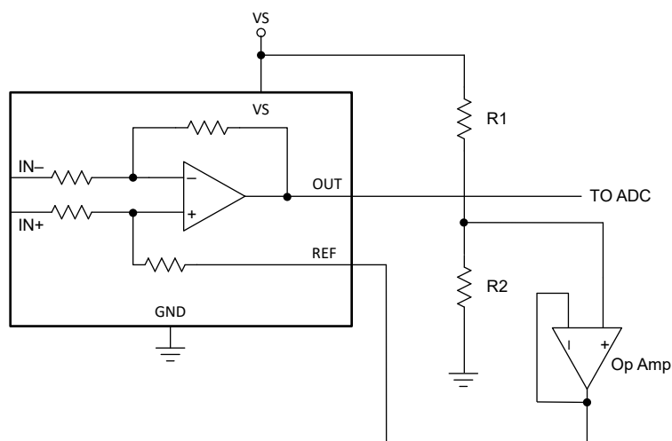
图 6-5. 1/2 V_s 电压输出
