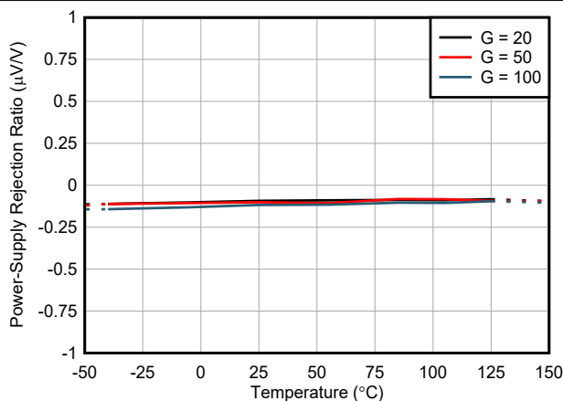
图 5-9. 电源抑制比与温度间的关系
