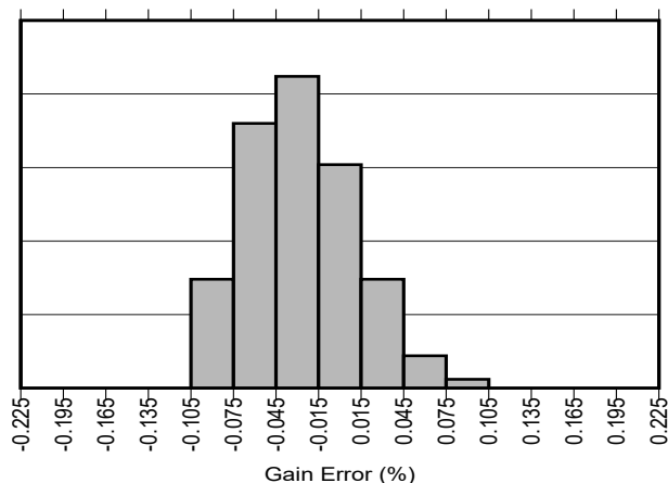
图 5-7. INA299-Q1 增益误差产生分布图
