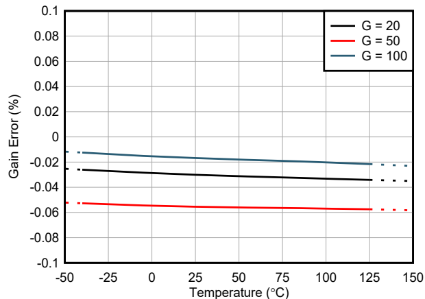
图 5-8. 增益误差与温度间的关系
