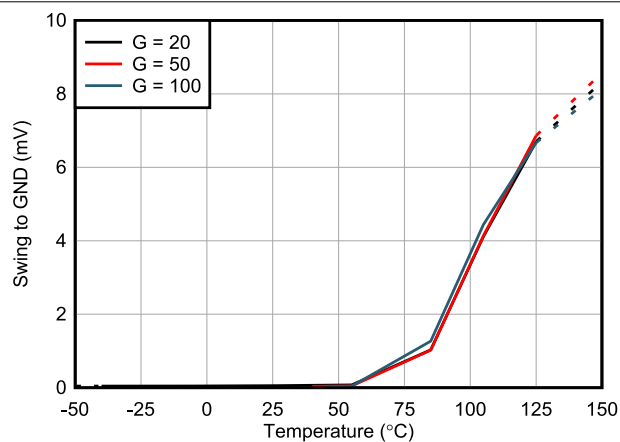
图 5-21. 相对于 GND 的摆幅与温度间的关系
