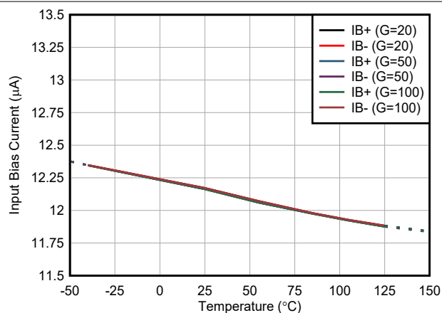
图 5-12. 输入偏置电流与温度间的关系
