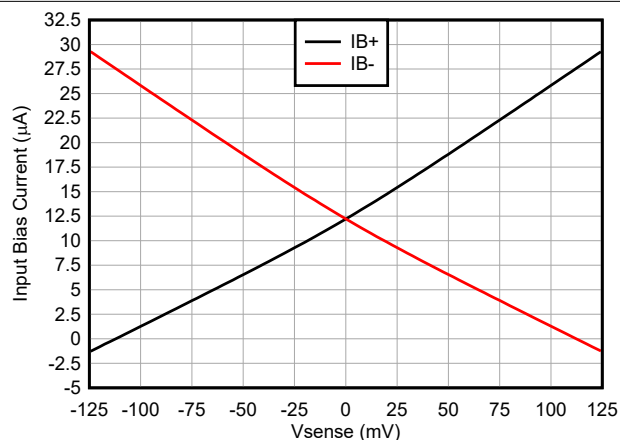
图 5-13. INA299-Q1 增益 = 20V/V，输入偏置电流与 V_{\text{SENSE}} 间的关系
