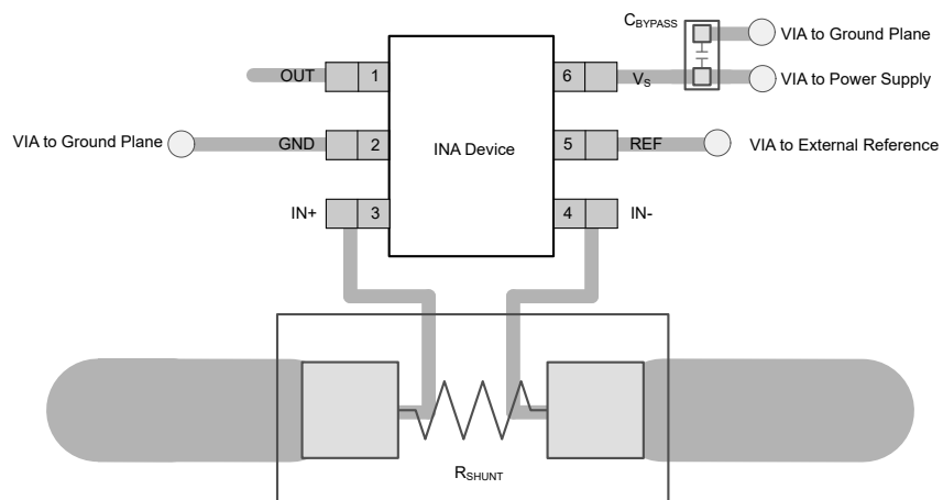
图 7-3. INA299-Q1 SOT-23 6 引脚 (DBV) 封装建议布局
