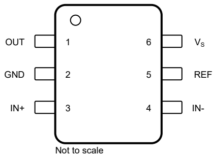
图 4-1. INA299-Q1 : DBV 封装 6 引脚 SOT-23 顶视图
