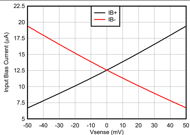
图 5-14. INA299-Q1 增益 = 50V/V，输入偏置电流与 V_{\text{SENSE}} 间的关系
