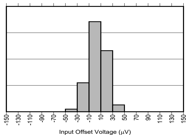
图 5-1. INA299-Q1 输入失调电压产生分布图
