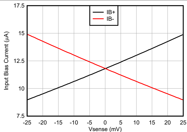
图 5-15. INA299-Q1 增益 = 100V/V，输入偏置电流与 V_{\text{SENSE}} 间的关系
