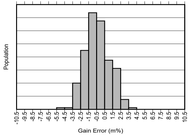
图 6-11. INA296A4-Q1 和 INA296A5-Q1 增益误差产生分布图
