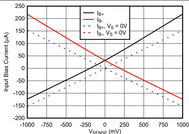
图 6-19. INA296x1-Q1 输入偏置电流与 V_{\text{SENSE}} 间的关系
