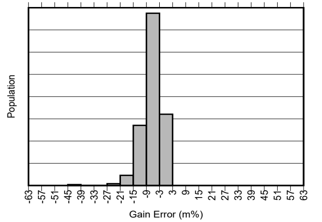
图 6-12. 所有增益 INA296B-Q1 增益误差产生分布图
