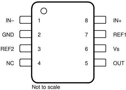
图 5-1. INA296x : DDF 封装 8 引脚 SOT-23 顶视图
