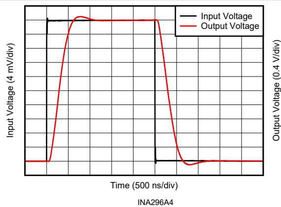
图 6-35. 大阶跃响应
