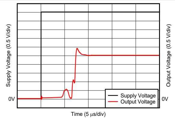
图 6-34. 小阶跃响应
