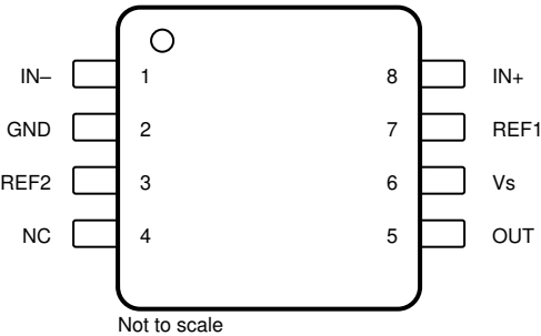
图 5-2. INA296x : D 和 DGK 封装 8 引脚 SOIC 和 8 引脚 VSSOP 顶视图
