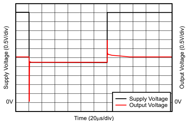
图 6-37. 欠压恢复
