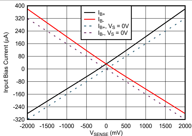
图 6-18. INA296x1-Q1 输入偏置电流与 V_{\text{SENSE}} 间的关系
