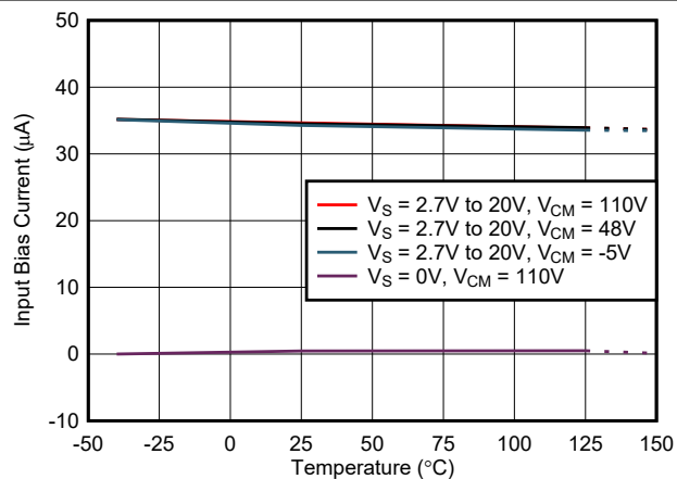
图 6-17. 输入偏置电流与温度间的关系
