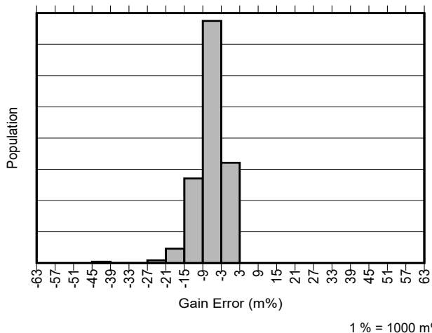
图 6-12. 所有增益 INA296B 增益误差产生分布图
