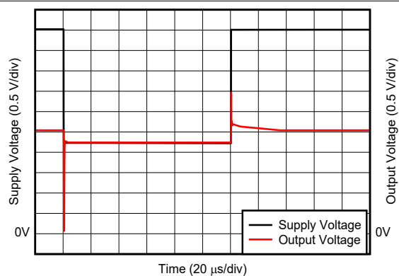
图 6-37. 欠压恢复
