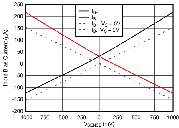
图 6-19. INA296x2 输入偏置电流与 V_{\text{SENSE}} 间的关系
