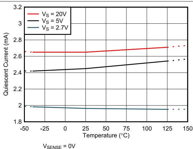
图 6-30. 静态电流与温度间的关系
