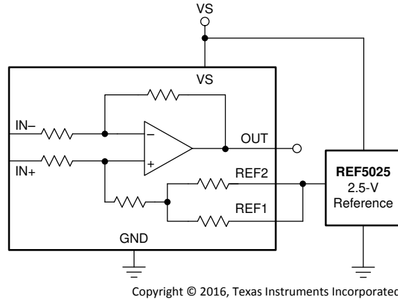
图 7-4. 外部基准输出
