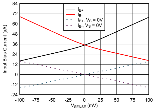
图 6-19. INA296x2 输入偏置电流与 V_{\text{SENSE}} 间的关系
