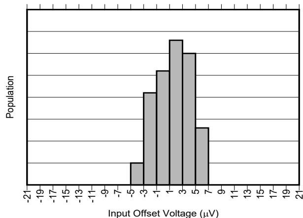
图 6-1. INA296A1 输入失调电压产生分布图
