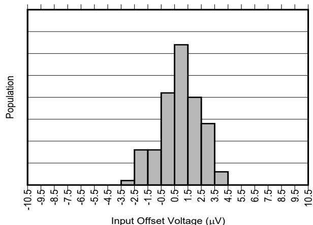
图 6-2. INA296A2 输入失调电压产生分布图
