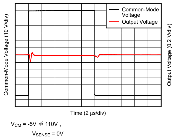
图 6-33. 共模电压快速瞬态脉冲
