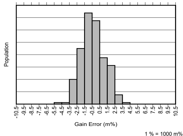
图 6-11. INA296A4 和 INA296A5 增益误差产生分布图
