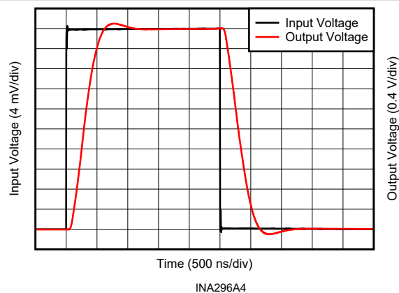
图 6-35. 大阶跃响应
