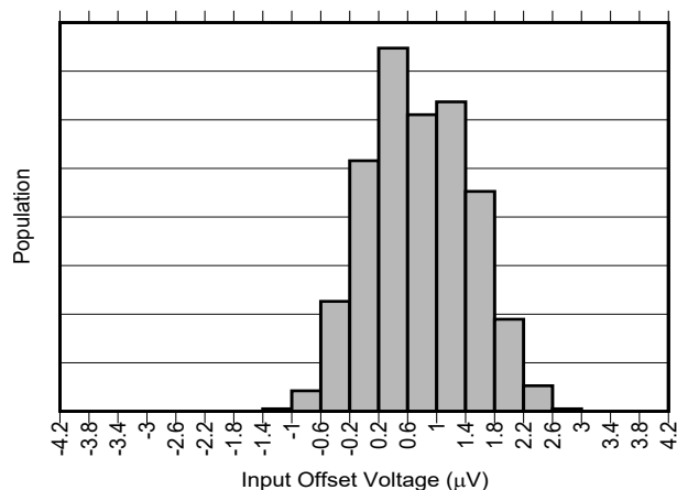
图 6-3. INA296A3 和 INA296A4 输入失调电压产生分布图
