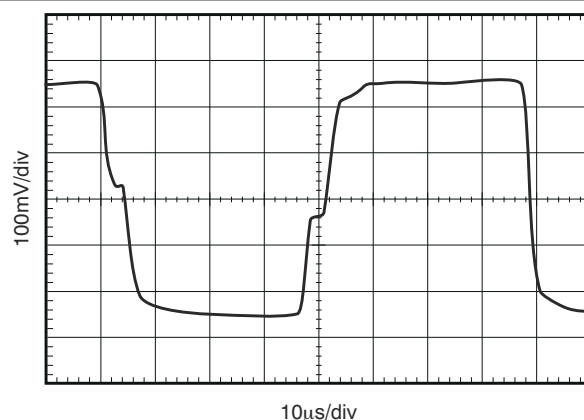
图 6-28. 500-mV Step Response
