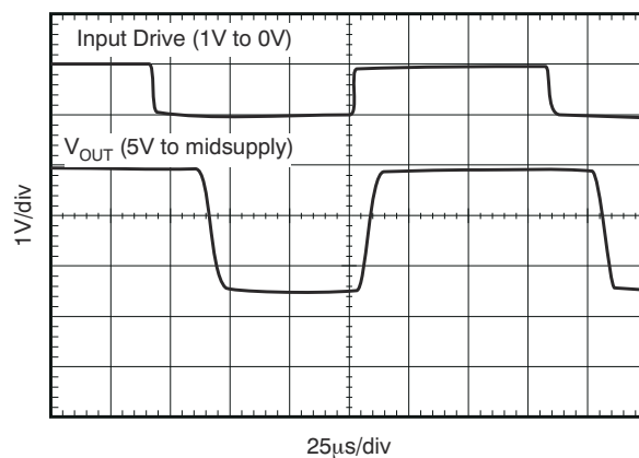
图 6-31. Input Overload
