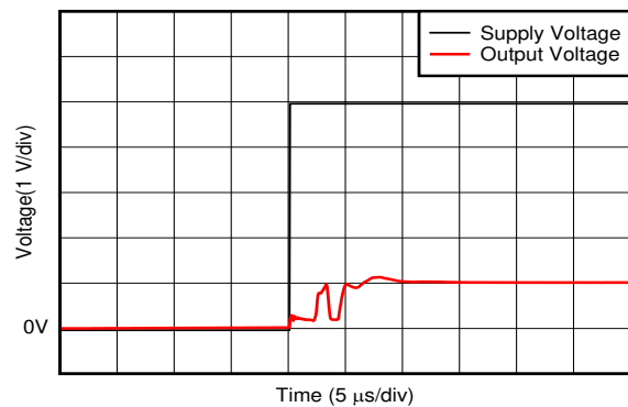
图 7-25. 启动响应
