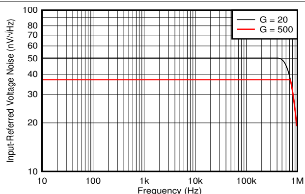
图 7-16. 输入参考噪声与频率间的关系
