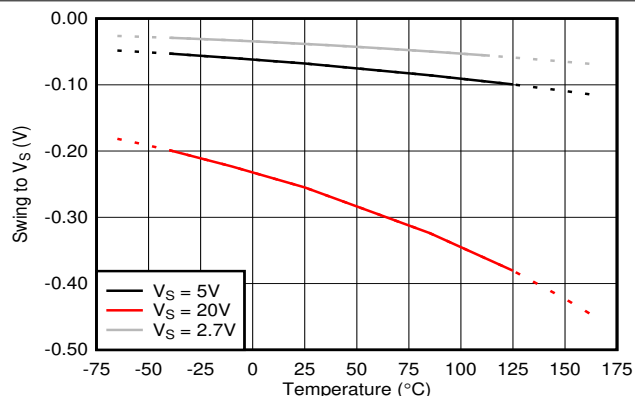
图 7-14. 电源摆幅与温度间的关系
