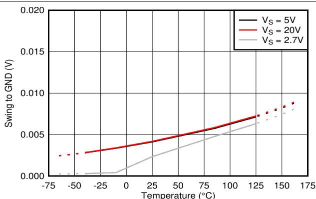
图 7-15. 相对于 GND 的摆幅与温度间的关系
