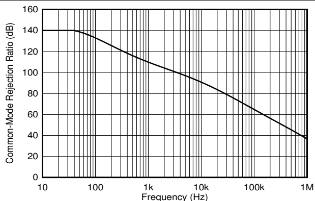
图 7-2. 共模抑制比与频率间的关系
