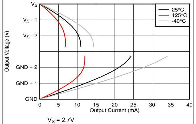
图 7-10. 输出电压与输出电流间的关系
