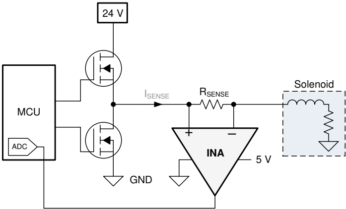
图 9-2. 螺线管应用中的电流检测
