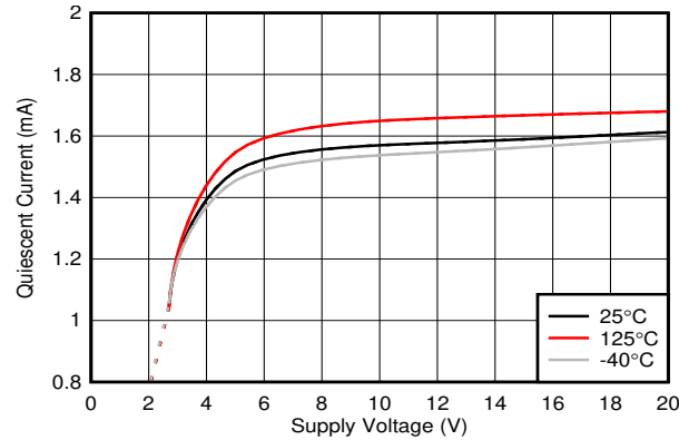
图 7-21. 静态电流与电源电压间的关系
