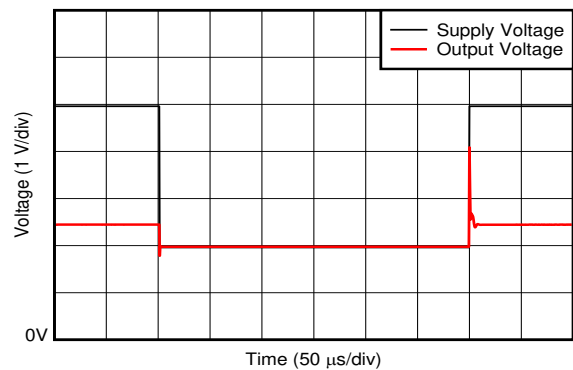
图 7-26. 电源瞬态响应
