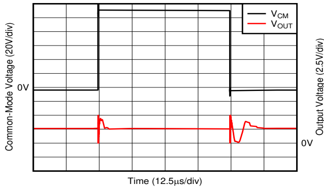
图 7-23. 共模电压快速瞬态脉冲
