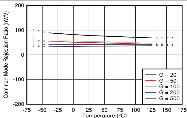
图 7-1. 共模抑制比与温度间的关系
