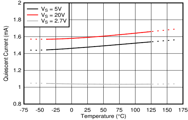
图 7-19. 静态电流与温度间的关系
