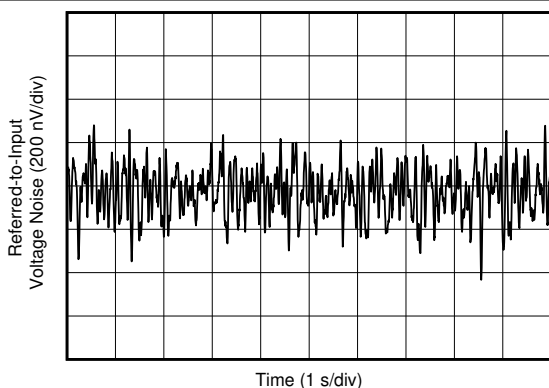
图 7-17. 输入参考噪声
