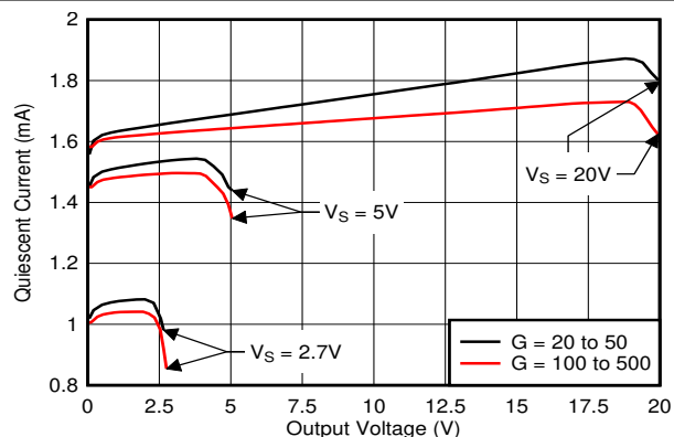
图 7-18. 静态电流与输出电压间的关系
