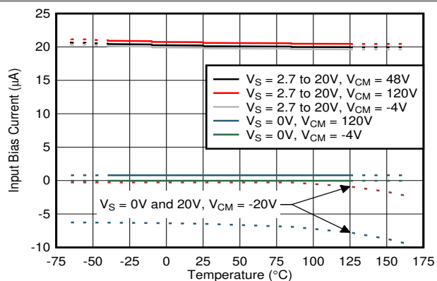
图 7-6. 输入偏置电流与温度间的关系
