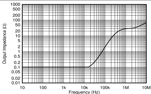
图 7-13. 输出阻抗与频率间的关系
