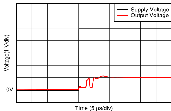
图 5-25. 启动响应
