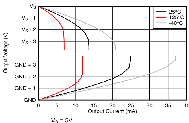
图 5-11. 输出电压与输出电流间的关系 V_S = 5\text{V}
