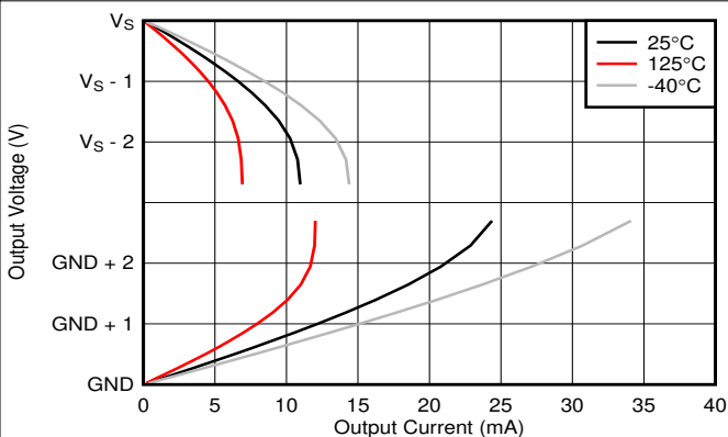
图 5-10. 输出电压与输出电流间的关系 V_S = 2.7\text{V}
