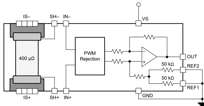
图 8-6. Ground-Referenced Output
