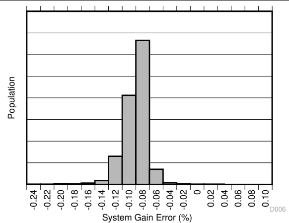
图 6-6. Gain Error Production Distribution (INA253A1-Q1)
