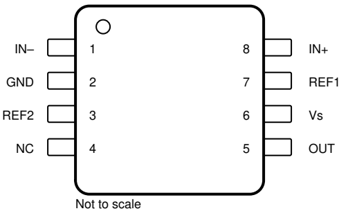
图 5-2. INA241x-Q1 : D 和 DGK 封装 8 引脚 SOIC 和 8 引脚 VSSOP 顶视图
