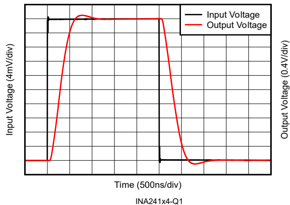
图 6-35. 大阶跃响应
