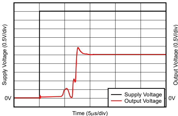
图 6-34. 小阶跃响应
