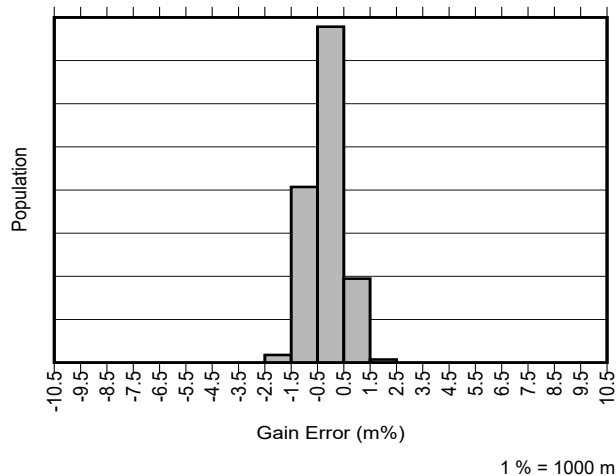
图 6-10. INA241A1-Q1, INA241A2-Q1, INA241A3-Q1 增益误差产生分布图
