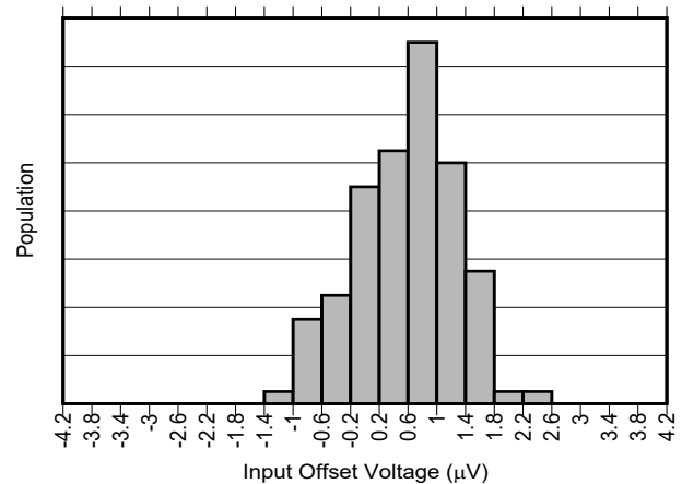
图 6-4. INA241A5-Q1 输入失调电压产生分布图
