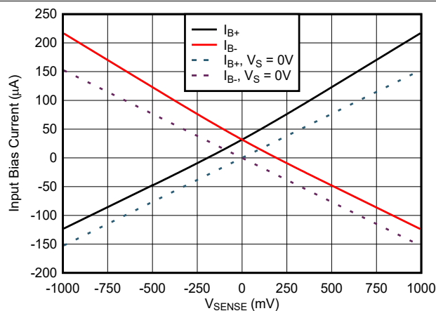
图 6-19. INA241x1-Q1 输入偏置电流与 V_{\text{SENSE}} 间的关系
