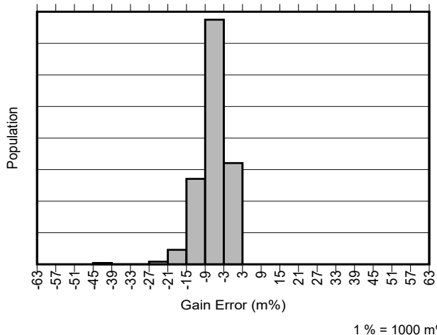
图 6-12. 所有增益 INA241B 增益误差产生分布图
