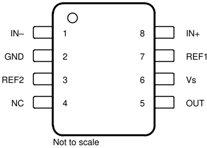
图 5-1. INA241x : DDF 封装 8 引脚 SOT-23 顶视图
