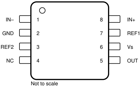
图 5-2. INA241x : D 和 DGK 封装 8 引脚 SOIC 和 8 引脚 VSSOP 顶视图
